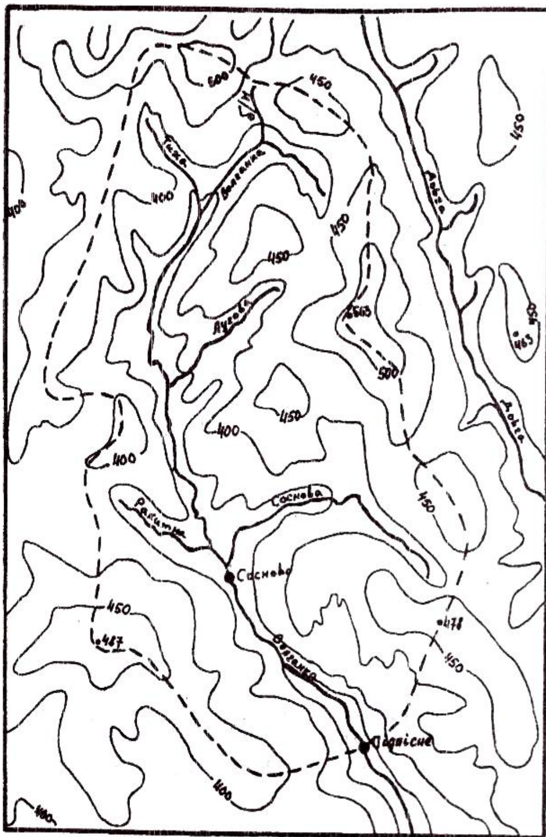
Рисунок 2.1 – Карта водозбору р. Волганки
