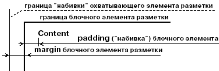
Рис. 3.7 Padding и margin – отступы блочного элемента
