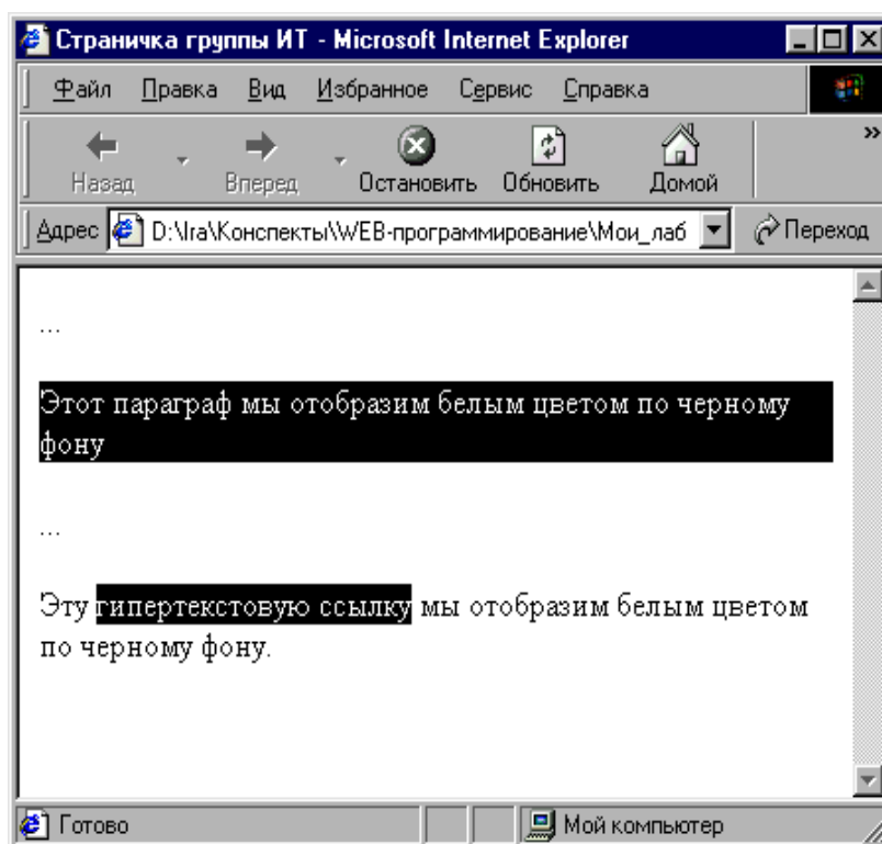
Рис.3. 2 Стиль белым цветом по черному фону
