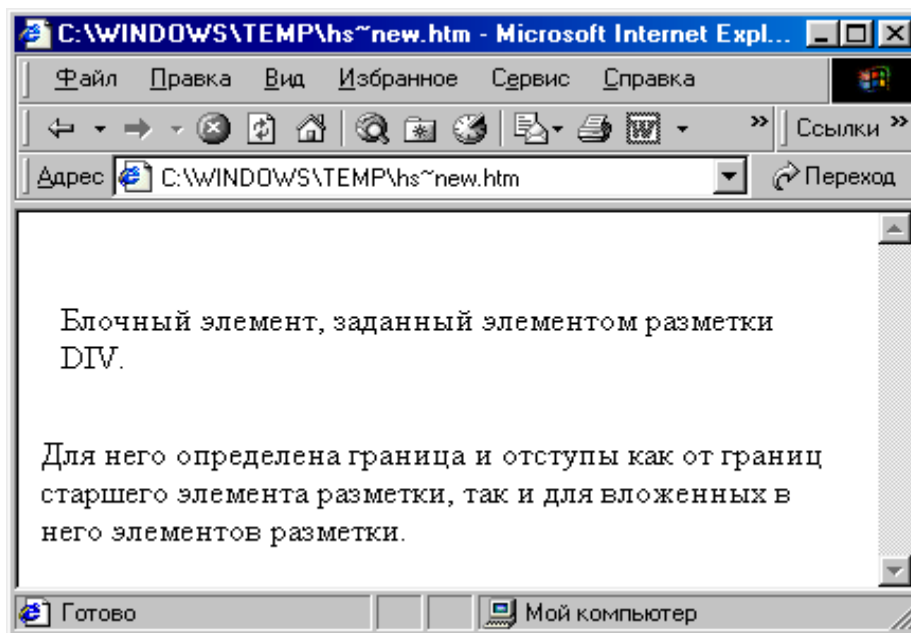
Рис.3. 10 Элемен разметки DIV
