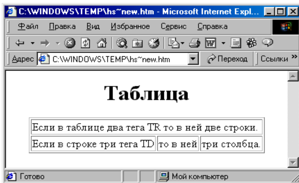
Рис. 2.3 Пример таблицы
