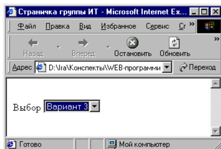
Рис.2.4 Пример формы
