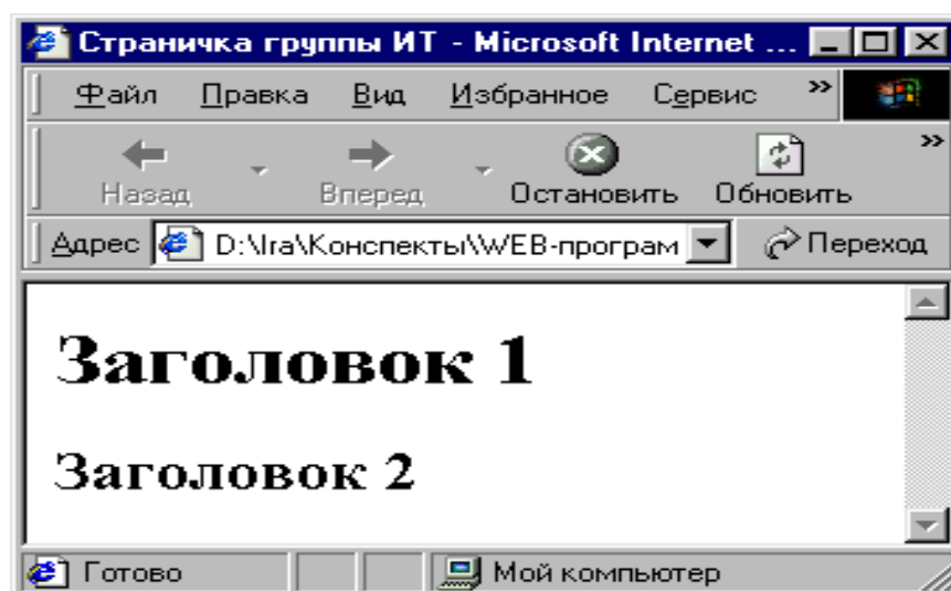
Рис.2.1 Заголовки
