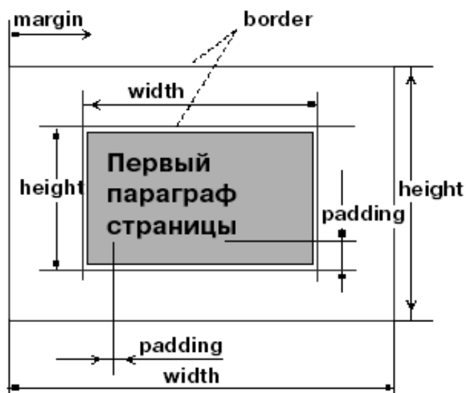
Рис. 3.11 Структура страницы
