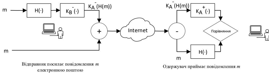
Рисунок 1.11 – Використання хеш-функції і цифрового підпису для аутентифікації і забезпечення цілісності повідомлення
