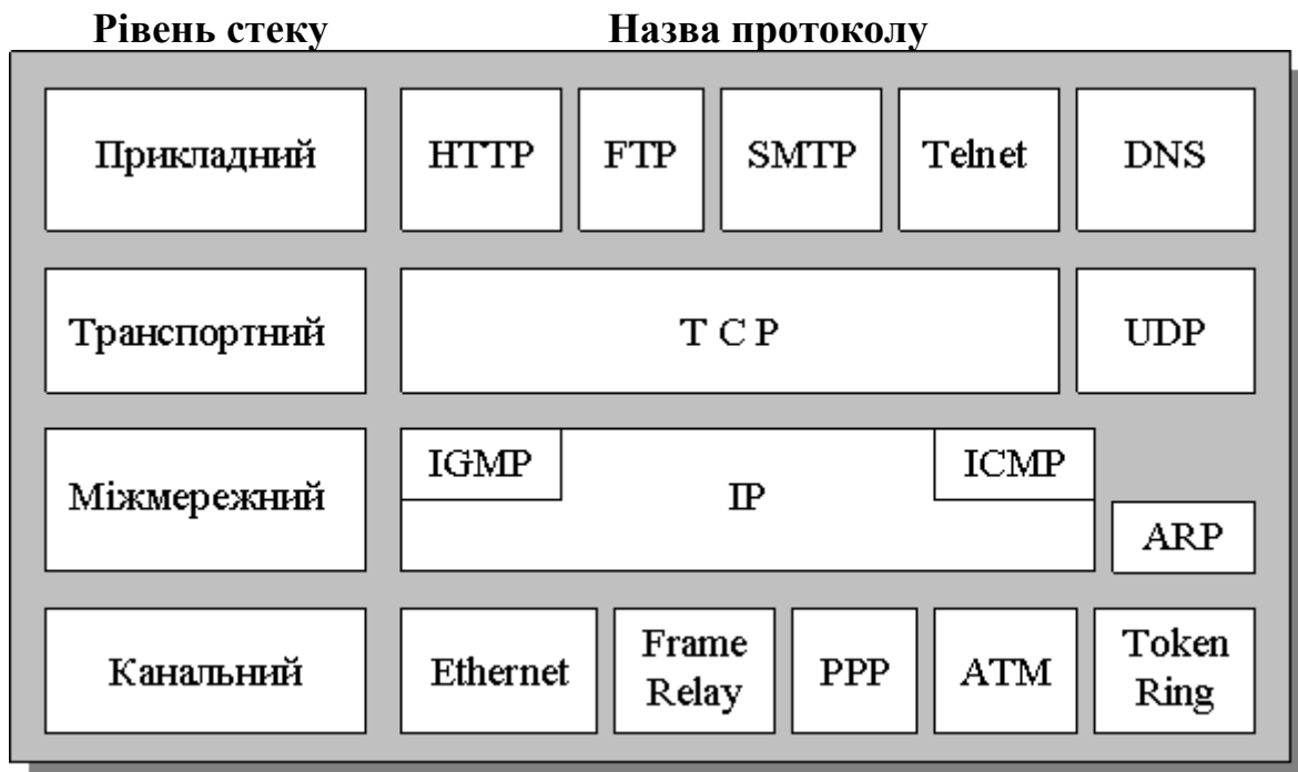
Рисунок 1.6 – Протоколи стеку TCP/IP
