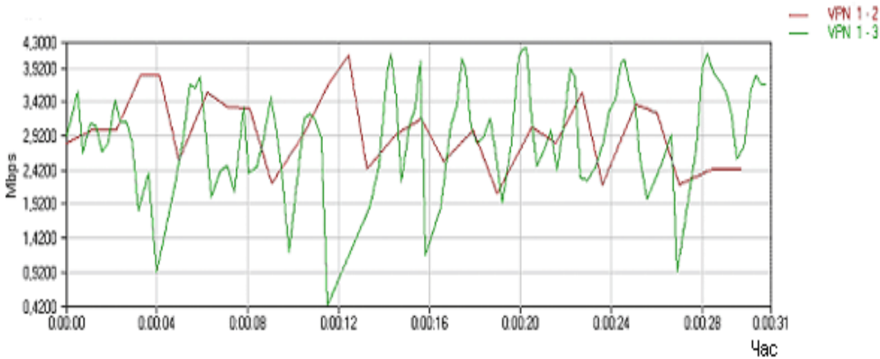
Рисунок 3.2 – Порівняння продуктивності VPN тунелів (1-2)
