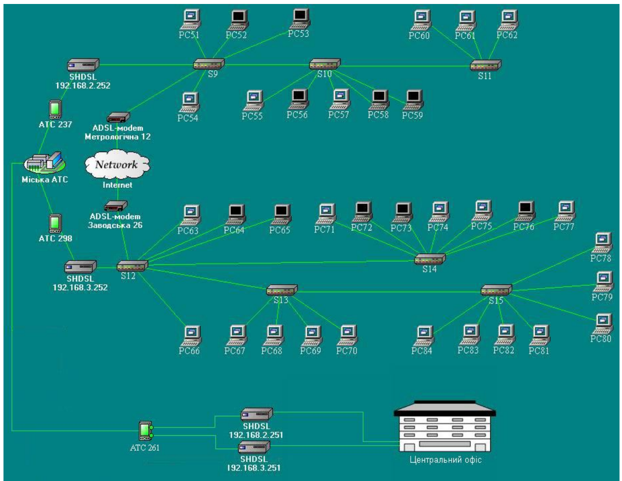
Рисунок 2.3 – Структура мережі київського відділу
