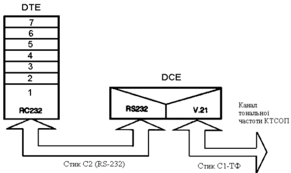
Рисунок 1.3 – Профіль протоколів для модема з функціями тільки фізичного рівня.
