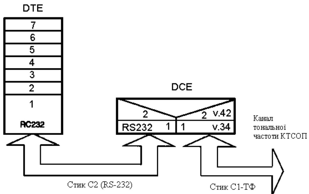
Рисунок 1.2 – Профіль протоколів для модема з функціями фізичного і каналного рівнів.
