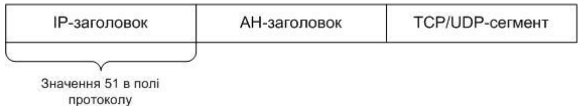
Рисунок 1.8 – Положення АН-заголовка в IP-дейтаграмі
