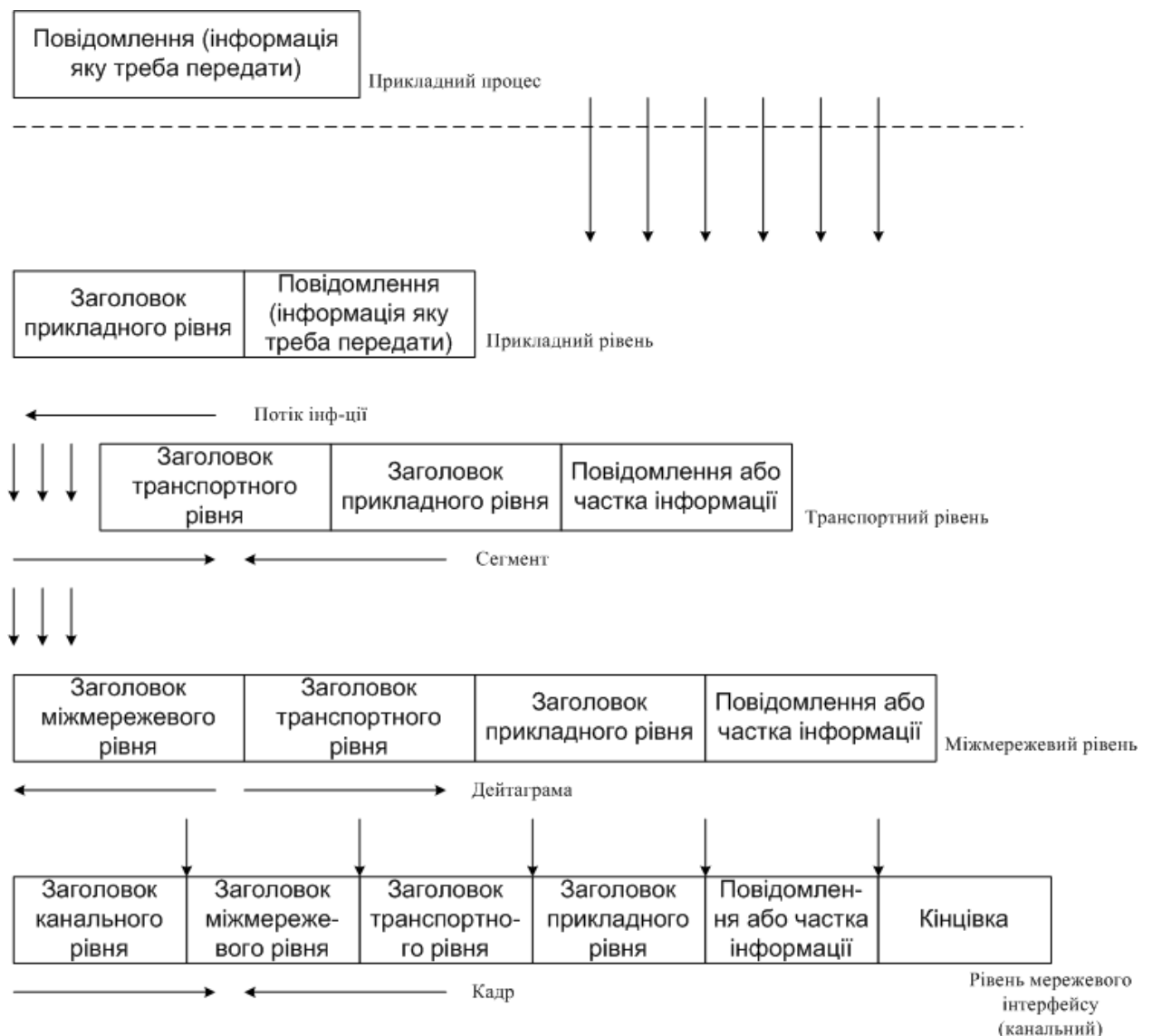
Рисунок 1.5 – Послідовність формування пакетів на ієрархічних рівнях стеку протоколів TCP/IP
