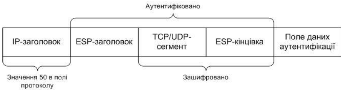
Рисунок 1.9 – Поля протоколу ESP в IP-дейтаграмі
