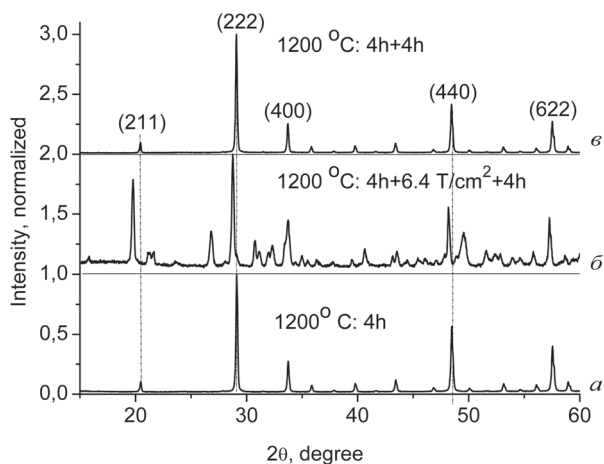
Дифракционные спектры Y_2O_3 : a – после отжига при 1200 °С в течение 4-х ч.; b – после предварительного отжига при 1200 °С в течение 4 ч, прессования при нагрузке 6,4 \times 10^3 кг/см 2 и дополнительного отжига при 1200 °С в течение 4 ч; c – образец после предварительного отжига при 1200 °С в течение 4 ч дополнительно отожжен при 1200 °С в течение 4 ч
