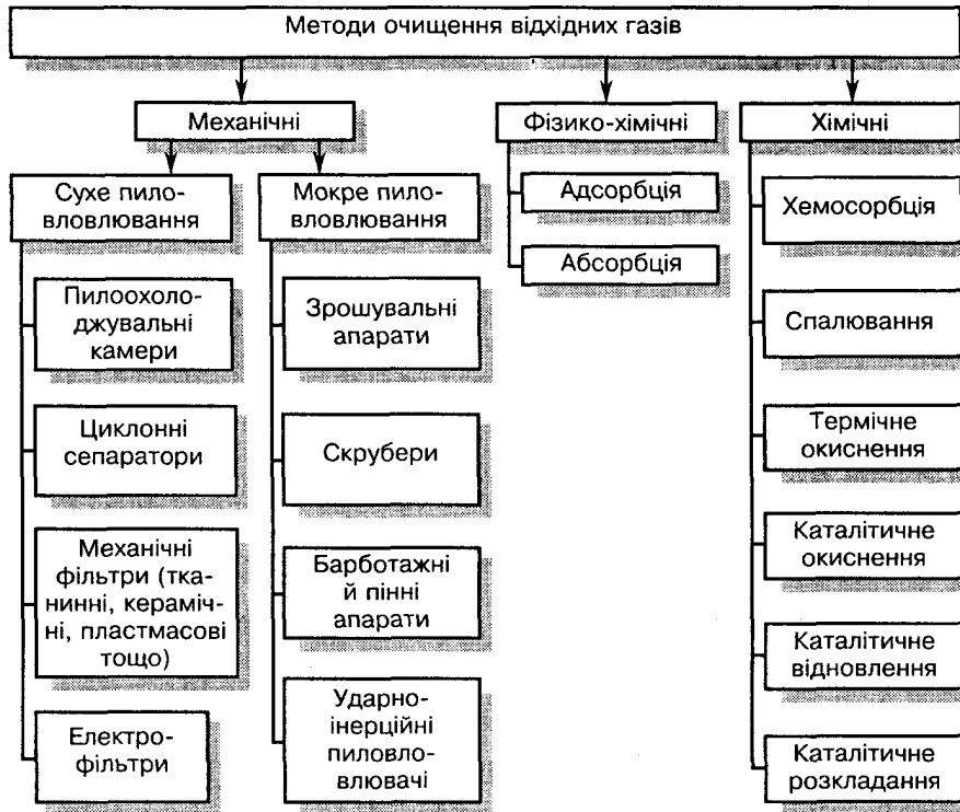
Рис. 1. Методи очищення газових викидів
