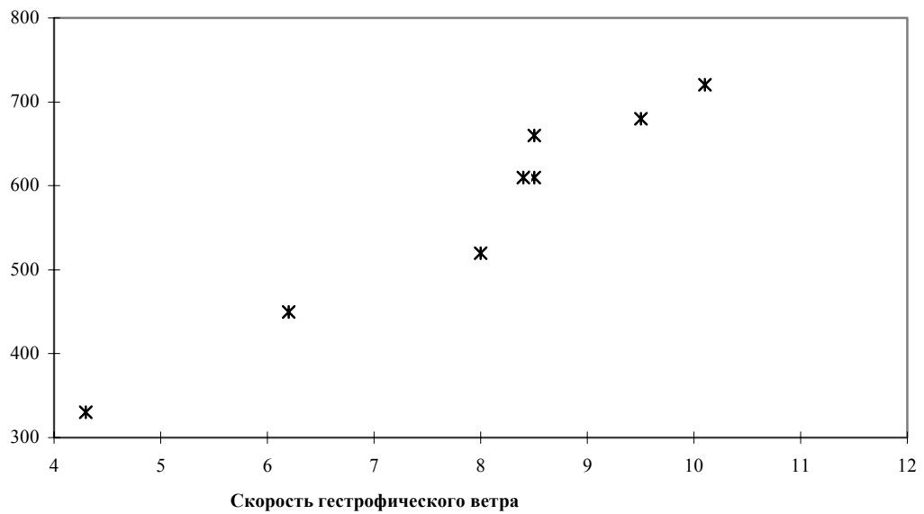
Рис. 6.3. Зависимость высоты АПС (м) от скорости невозмущенного потока (м/с) для климатических классов
