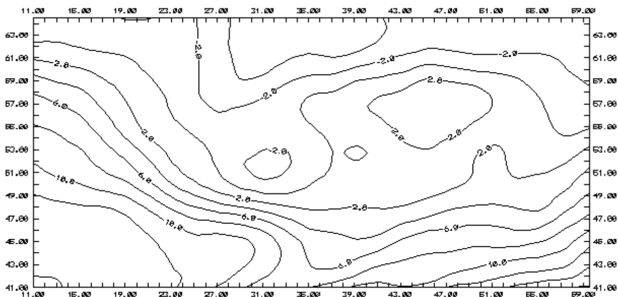
Рис. 4.6. Поле температуры на уровне 850 гПа за 06.10.97г., 00 час. СГВ
