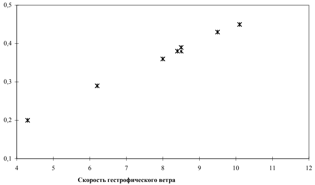
Рис. 6.2. Зависимость V_* (м/с) от скорости невозмущенного потока (м/с) для климатических классов
