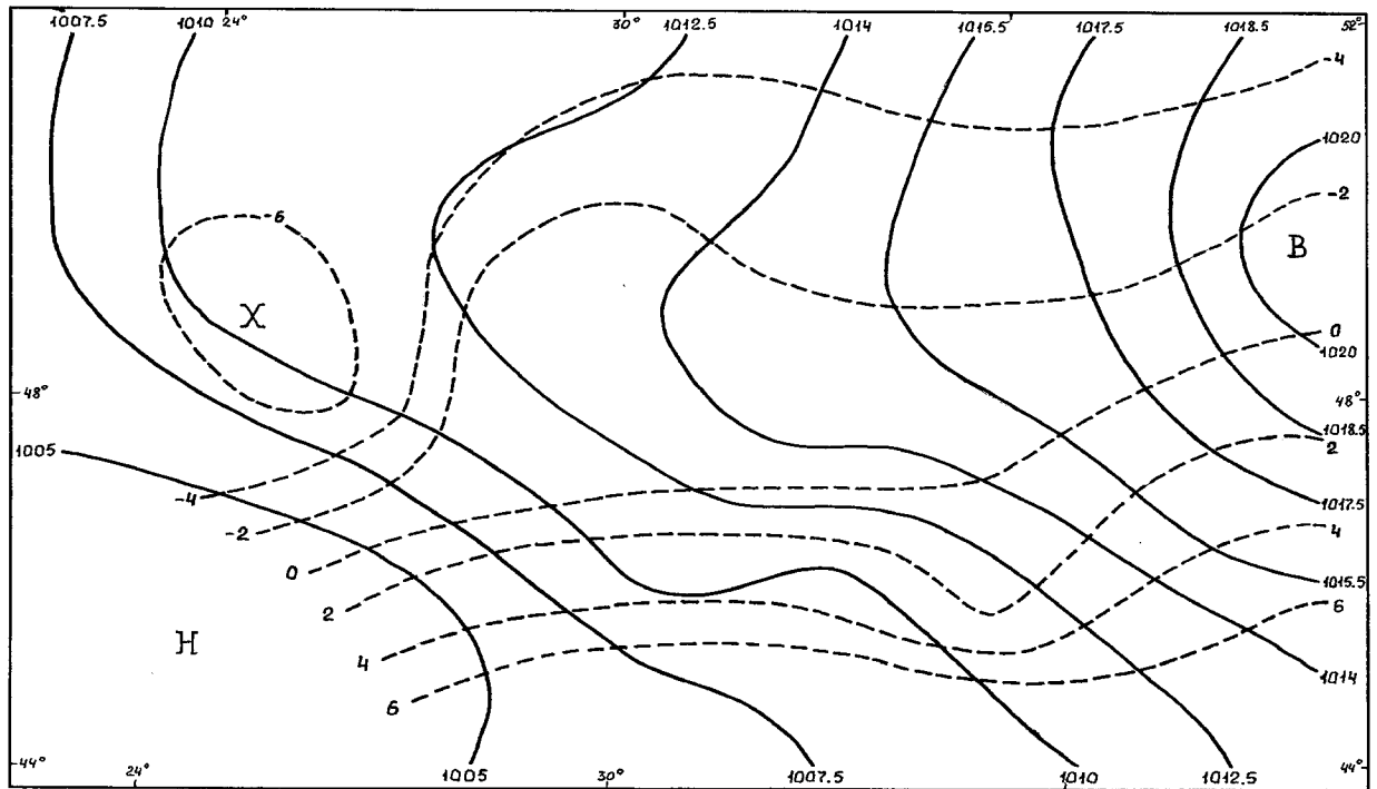
Рис. 3.1. Термобарическое поле у Земли над Украиной 07.01.86г., 12 час СГВ Обозначения: Сплошные линии - изобары, пунктирные линии - изотермы
