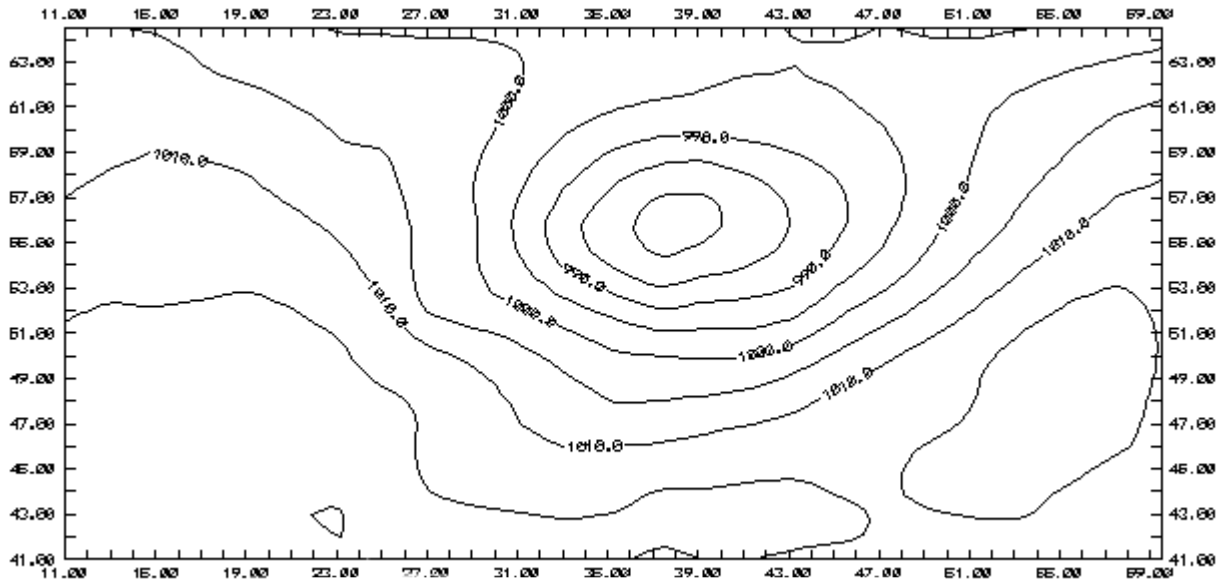
Рис. 3.32. Приземное поле давления за 06.10.97г., 00 час СГВ
