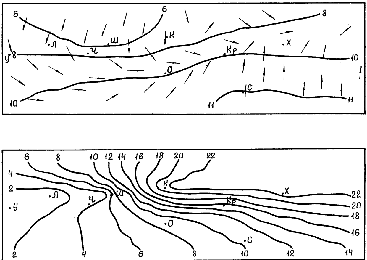
Рис. 3.23. Распределение характеристик внутренней структуры АПС на высоте 200 м за 23.05.87г., 12 час СВВ (обозначения см. рис.3.4)
