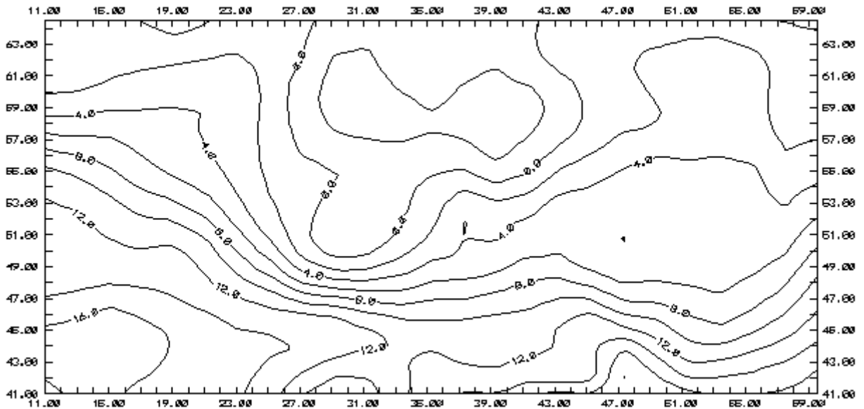
Рис. 3.36. Поле температуры на уровне 925 гПа за 06.10.97г., 00 час СГВ
