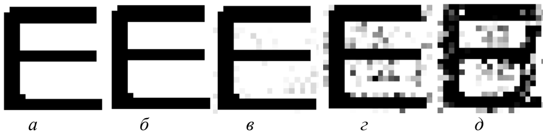
Рис. 2.8 – Результат розпізнавання навченою штучною нейронною мережею Хопфілда зашумленої букви Е: a - 0.0 , б - 0.1 , в - 0.5 , г - 1.5 , д - 2.5
