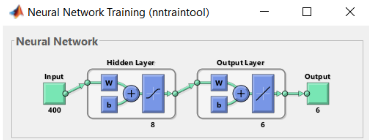
Рис. 2.2 – Архітектура створеної штучної нейронної мережі прямого поширення сигналу з одним прихованим шаром
