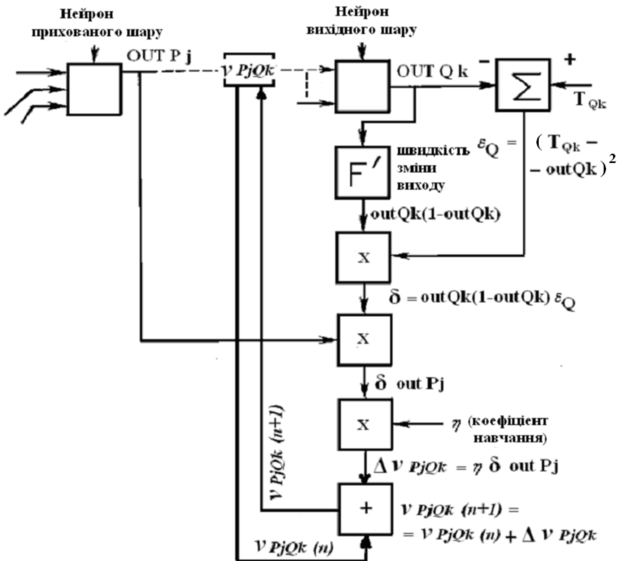
Рис. 1.3 – Налаштування вагів вихідного шару
