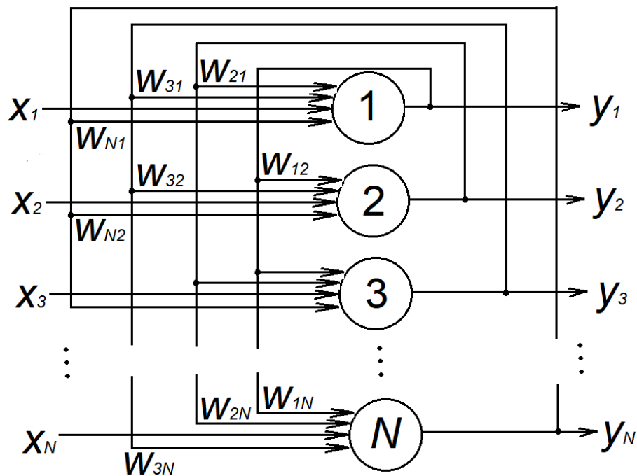
Рис. 1.6 – Структурна схема мережі Хопфілда
