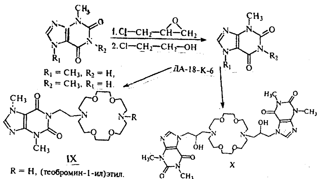
Схема 2 – Конденсация галогеналкил- и эпоксиалкилпуринов.
