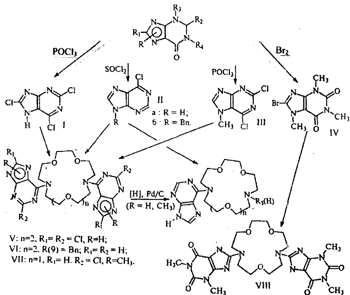
Схема 1 – Синтез краун-пуринов на основе галогенпуринов
