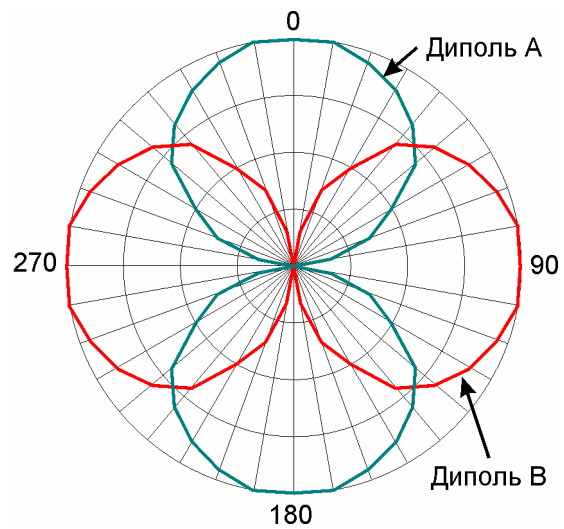
Рис. 3.4 – Діаграма направленості антени в горизонтальній площині
