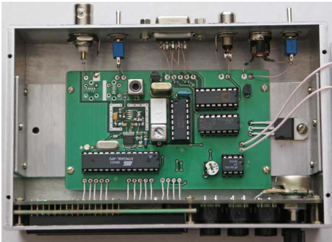
Рис. 3.14 – Вигляд приймача з боку розташування деталей
