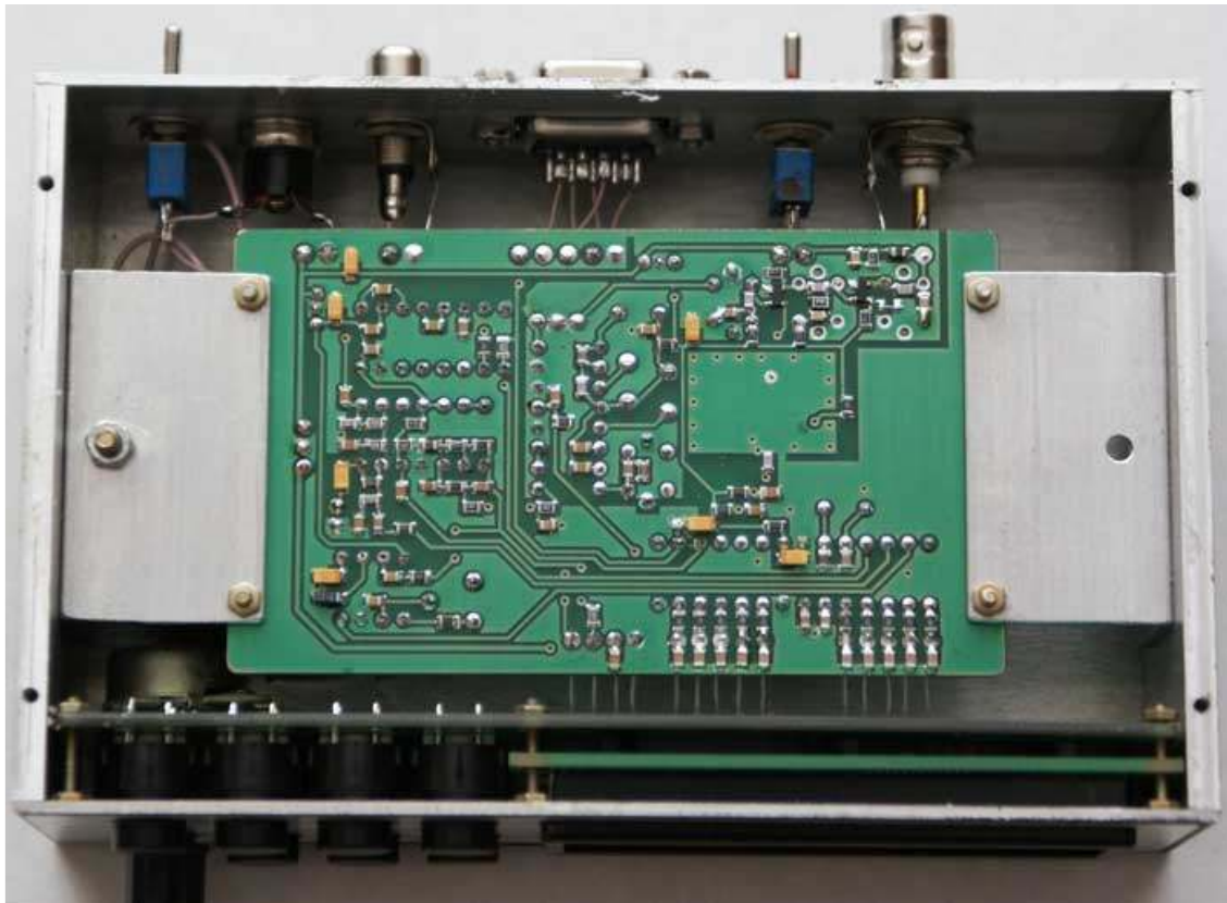
Рис. 3.15 – Вигляд приймача з боку друкарського монтажу
