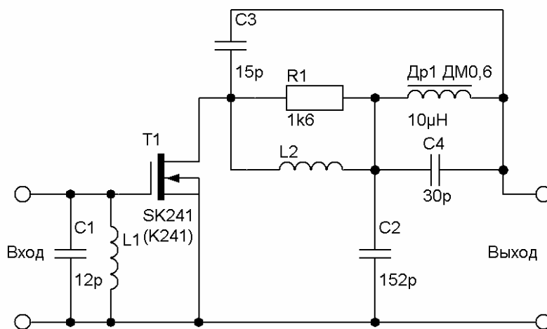
Рис. 3.10 – Принципова схема антенного підсилювача
