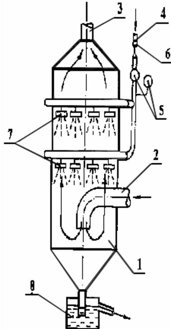
Рисунок 4 .1 – Скрубер з форсунками (1- циліндричний корпус, 2- вхідний патрубок, 3 - патрубок для відводу газу, який очищено, 4 – підвід води для зрошення , 5 – контрольні-вимірні прилади параметрів води, 6- регульована засувка, 7 – форсунки верхнього та нижнього ярусів зрошення, 8 – гідрозатвор)
