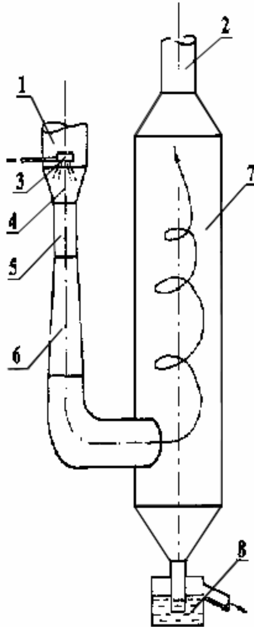
Рисунок 4.4 - Скрубер Вентурі ( 1 - вхід газу, який потрібно очистити, 2 - вихід очищеного газу, 3 - пристрій для зрошення, 4 - конфузур труби Вентурі, 5 - горловина, 6 - дифузор, 7 - краплиноуловлювач, 8 – гідрозатвор)
