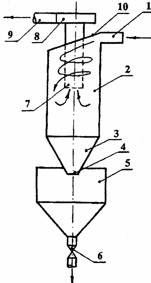
Рис. 3.2 – Циклон ( 1- вхідний патрубок , 2 – циліндрична частина корпусу, 3 – конічна частина корпусу, 4 – пиловипускний отвір, 5 – бункер для пилу, 6 – пиловий затвор, 7 – вихлопна труба, 8 – равлик, що розкручує повітря, 9 – вихідний патрубок, 10 – кришка під нахилом)
