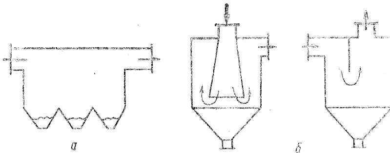
Рисунок 3.1 - Основні типи пилоосаджувальних камер
