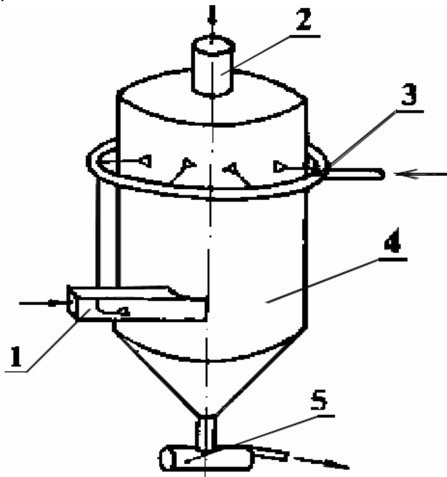
Рисунок 4.3 – Відцентровий скрубер ( 1 – тангенціальний патрубок для входу газу, який потрібно очистити, 2 – вихід очищеного газу, 3 – система подавання води, 4 – циліндричний корпус, 5 – гідрозатвор)
