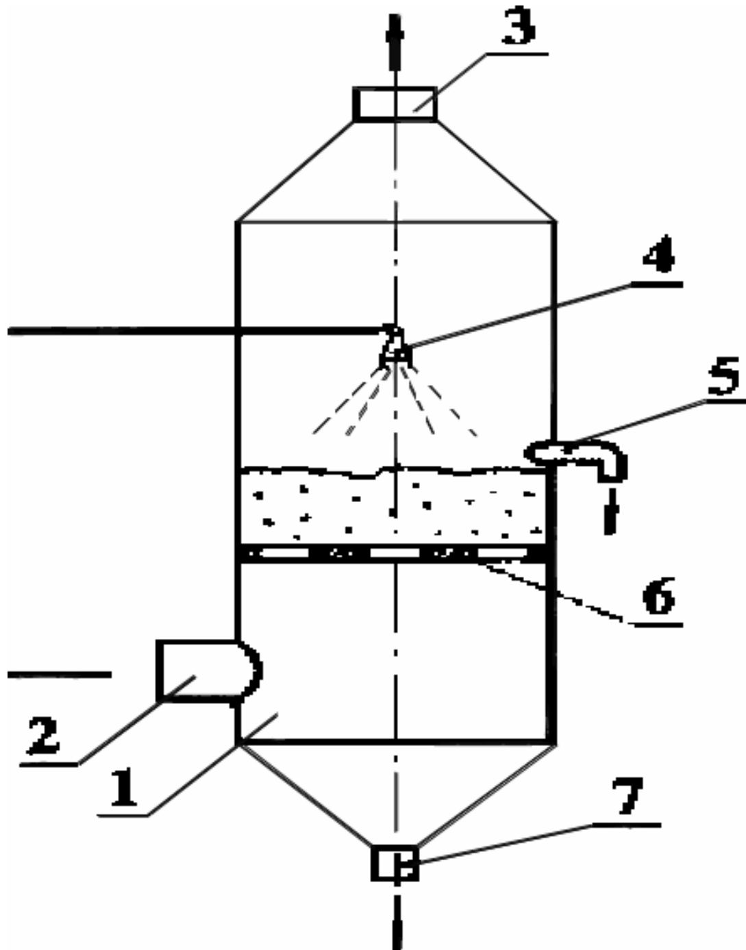
Рисунок 4.2 – Барбота́жний пінний апарат ( 1- корпус, 2- вхід повітря, 3 – вихід очищеного газу , 4 – зрошувач, 5 – відвід рідини у переливний відсік, 6 – решітка, 7 – відвід рідини, яка пройшла через решітку)
