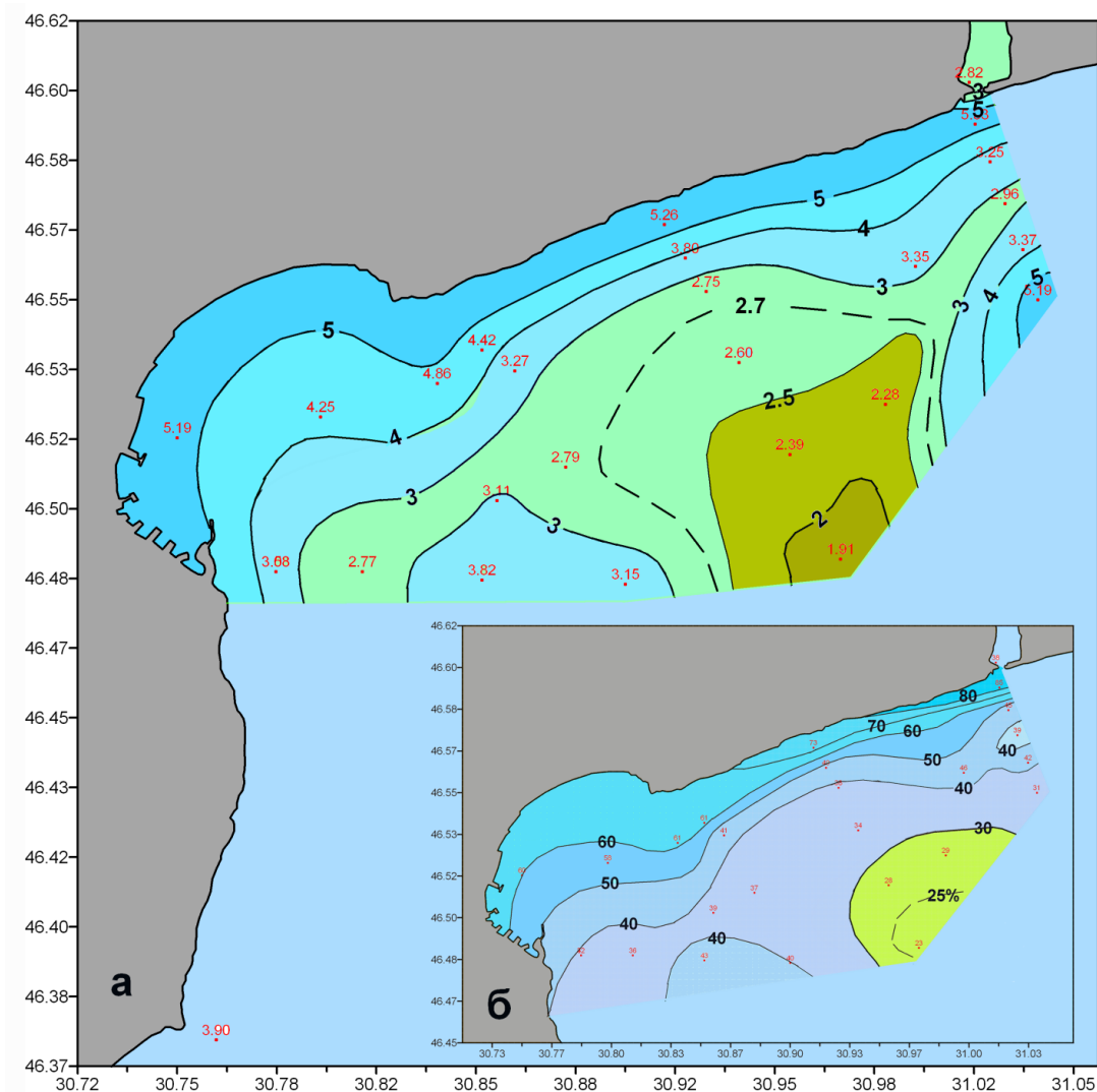
Рис. 1. Распределение растворенного кислорода (а – [мл·л -1 ], б – % насыщения) в придонном слое на северо-западном шельфе Черного моря
