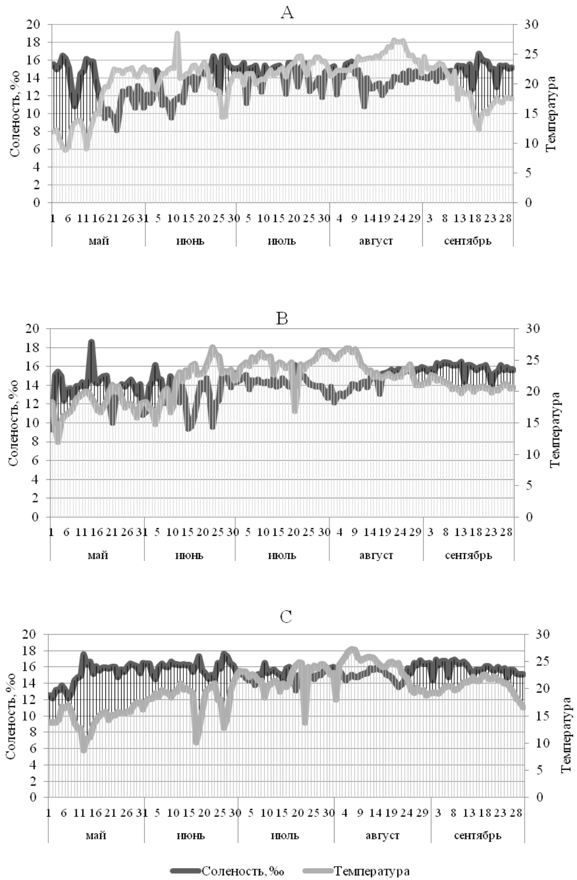
Рис. 2. Среднесуточные значения температуры и солености на поверхности моря (А - май - сентябрь, 2007; В - май - сентябрь, 2012; С - май - сентябрь, 2017).
