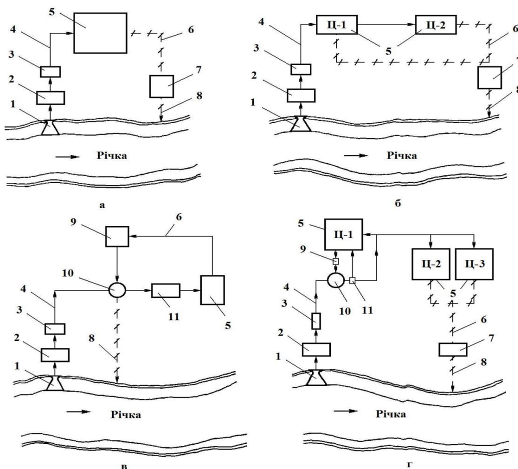
Рис. 2.1 – Схеми промислового водопостачання:
