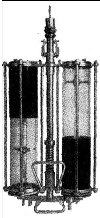
Рис. 4.4 – Батометр Молчанова ГР-18
