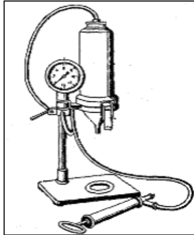
Рис. 4.5 – Прилад для примусової фільтрації (прилад Куприна) ГР-60
