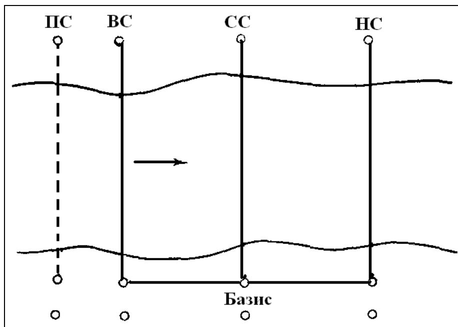
Рис. 3.1 – Схема розташування створів для вимірювання витрати води поверхневими поплавцями: ПС – пусковий ствір, ВС – верхній ствір, СС – середній ствір, НС – нижній ствір
