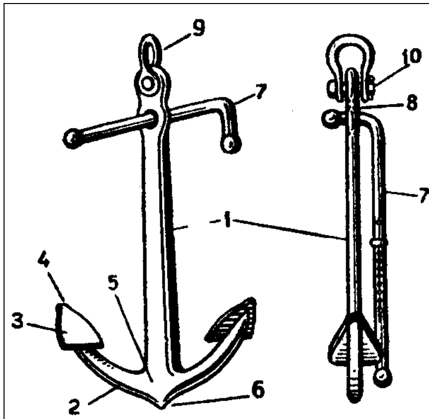
Рис. А.1 – Адміралтейський якір: 1 – веретено; 2 – ріг; 3 – лапа; 4 – носок; 5 – тренд; 6 – п'ятка; 7 – шток; 8 – шийка; 9 – скоба; 10 – болт
