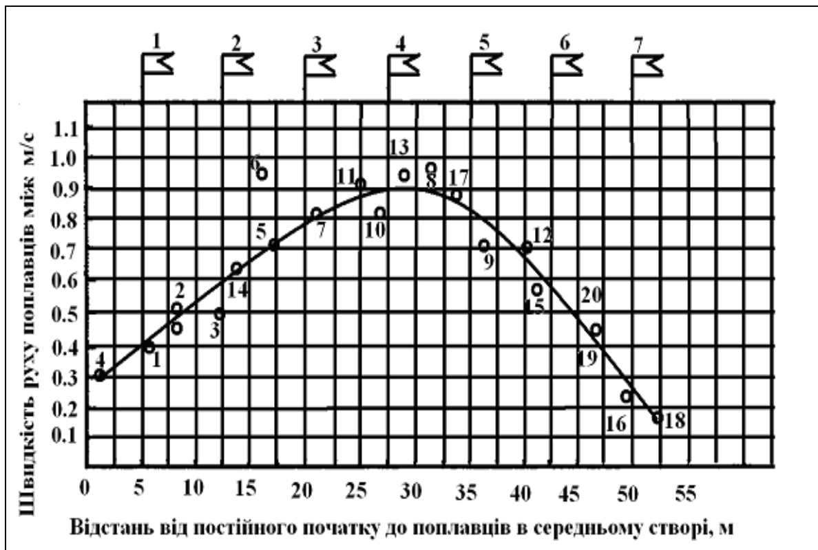
Рис. 3.2 – Епюра розподілу швидкості руху поплавців по ширині річки
