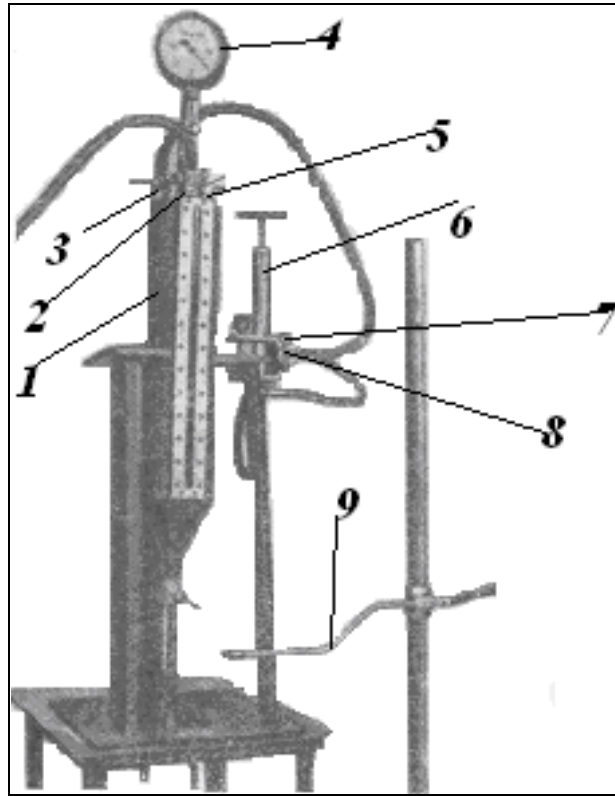
Рис. 4.1 – Батометр вакуумний ГР-61:
