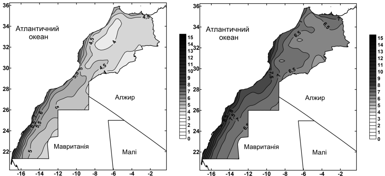
Рис. 1: а – середня за ансамблем моделей середньорічна швидкість вітру (м/с); б – середній за ансамблем моделей добовий максимум швидкості вітру (м/с) для періоду 2020–2050 рр.
