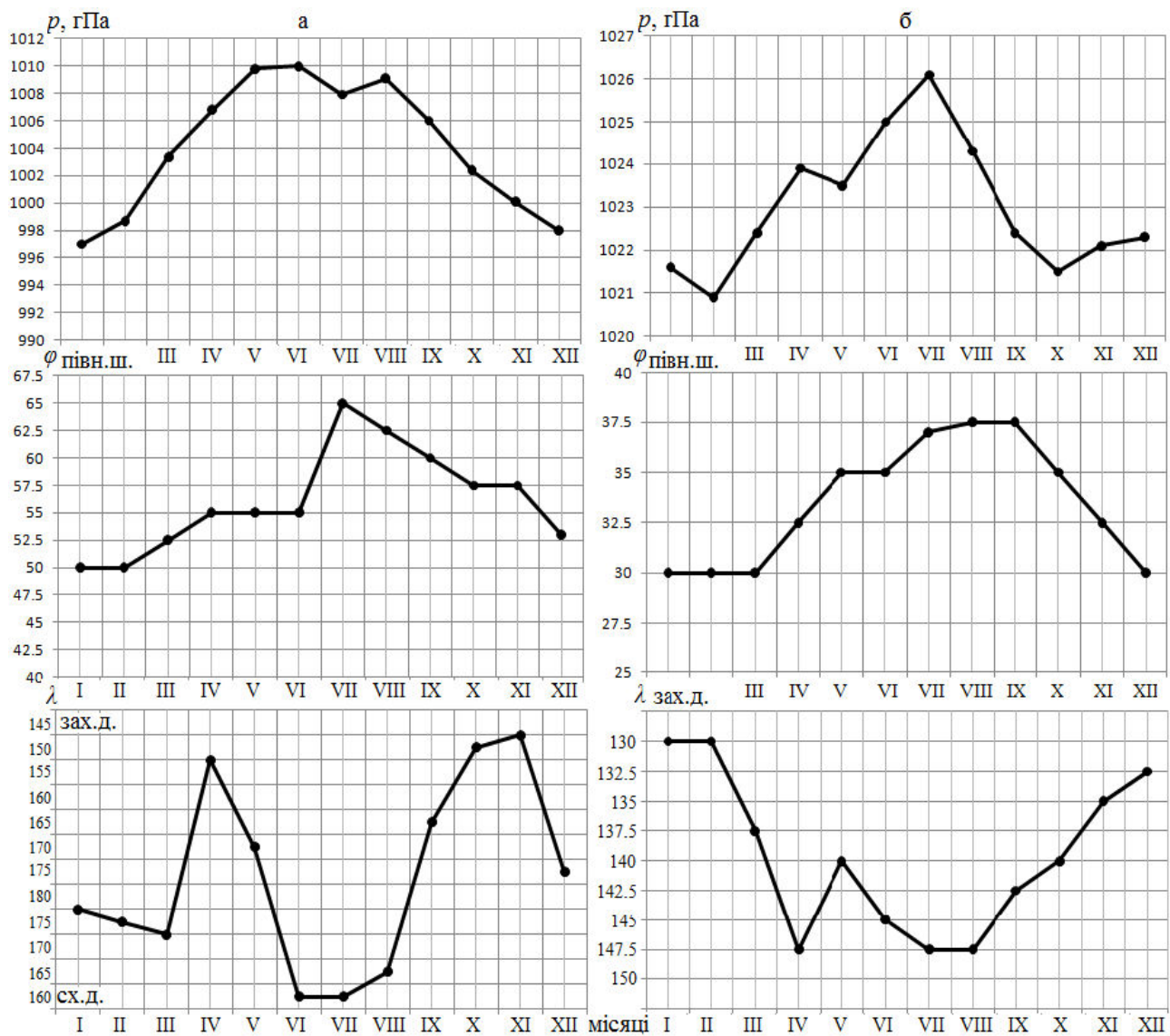
Рис. 1 – Сезонні зміни тиску, широти й довготи центрів дії атмосфери в північній частині Тихого океану: алеутська депресія (а); гонолульський максимум (б).
