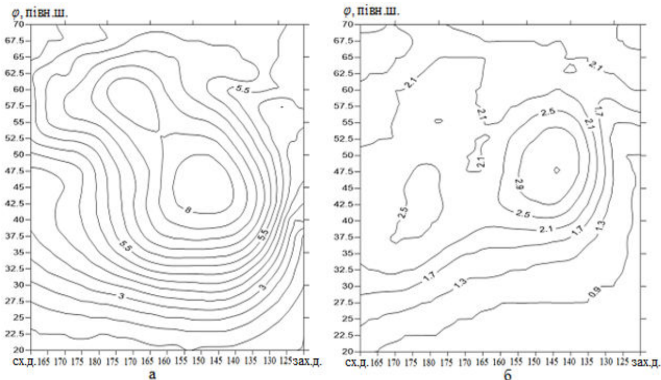
Рис. 2 – Поля середніх квадратичних відхилень приземного атмосферного тиску в січні (а) та липні (б).
