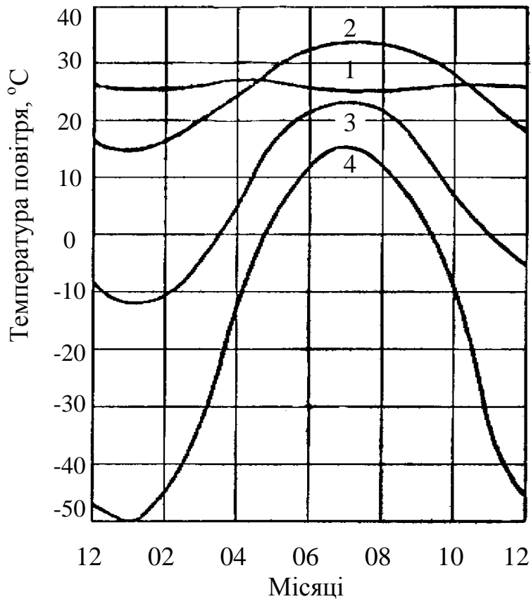
Рис. 5.2 – Типи річного ходу температури повітря: 1 – екваторіальний (Джакарта, \varphi = 6^{\circ} півд. шир.); 2 – тропічний (Асуан, \varphi = 24^{\circ} півн. шир.); 3 – помірного поясу (Саратов, \varphi = 52^{\circ} півн. ш.); 4 – полярний (Верхоянськ, \varphi = 67^{\circ} півн. ш.).
