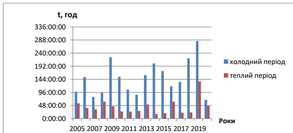
Рисунок 2 – Графік тривалості туманів на АМСЦ Херсон за теплий та холодний періоди (2005-2020 рр.)
