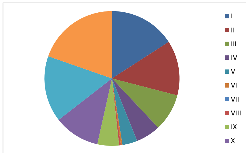
Рисунок 1 – Імовірність туману в холодний і теплий період на АМСЦ Херсон по місяцях (%)
