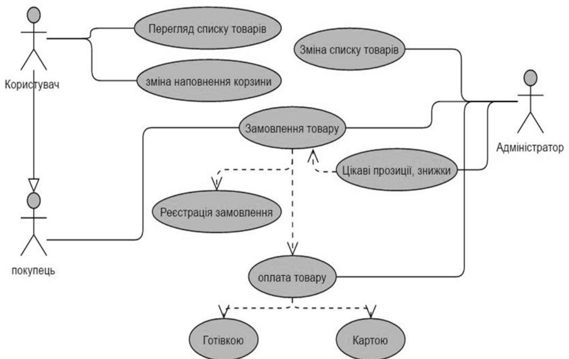
Рисунок 3.3 – Use Case діаграма
