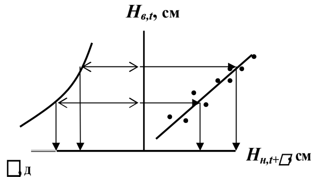
Рис.8.7 – Графік відповідних рівнів води при \Delta \neq \text{const}
