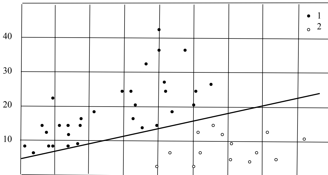
Рис.12.1 – Залежність \sum \square_{-min} = f(\square_0)
