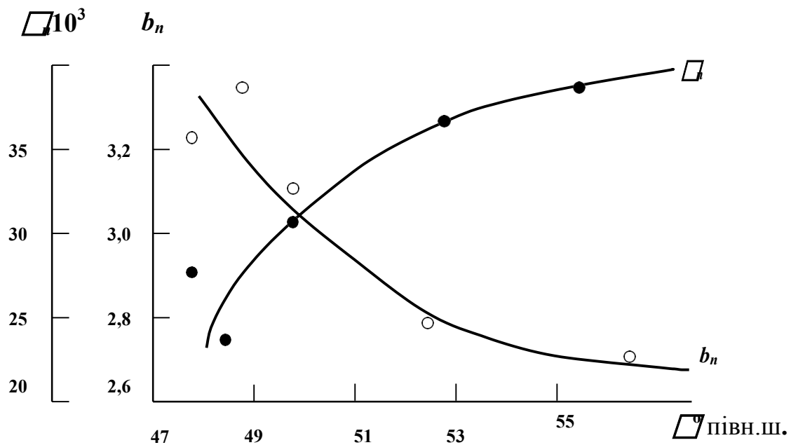
Рис.11.1 - Зміна коефіцієнтів \gamma_n і b_n в залежності від широти місцевості
