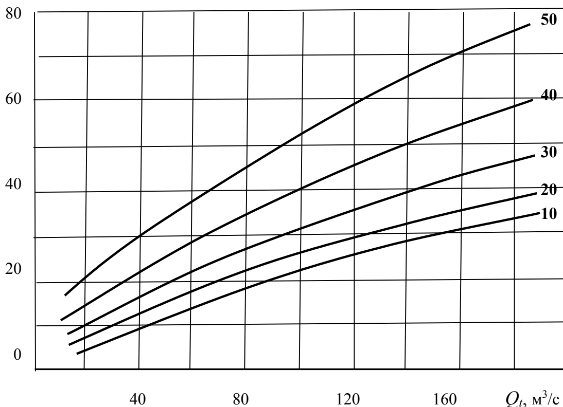
Рис. 10.2 – Загальний вигляд залежності місячного стоку літньо-осіннього періоду ( \bar{Q}_{t+30} ) від витрати води в початковий момент часу ( Q_t ) і кількості опадів ( X )
