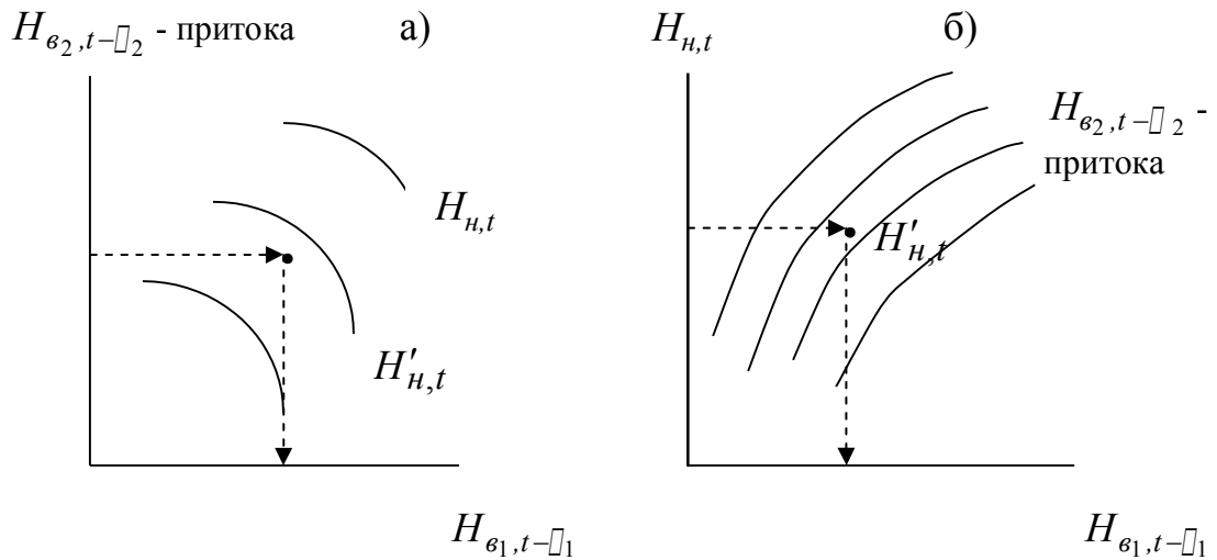
Рис. 8.13 – Приклади розробки методики прогнозу рівнів води за методом відповідних витрат (рівнів) води на припливних ділянках річок при \tau_1 \neq \tau_2
