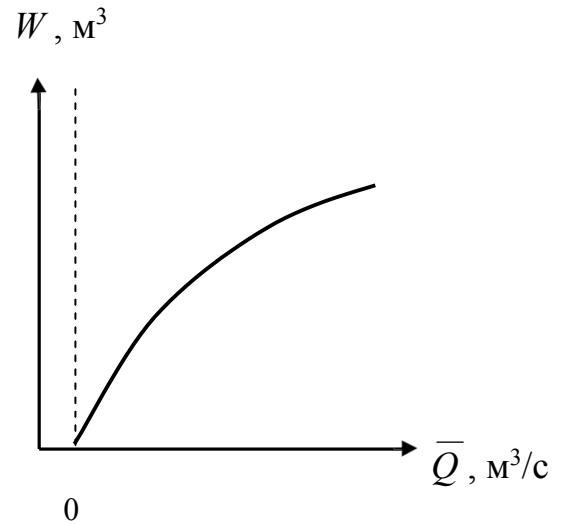
Рис. 9.5 - Типова крива руслових запасів води на ділянці річки
