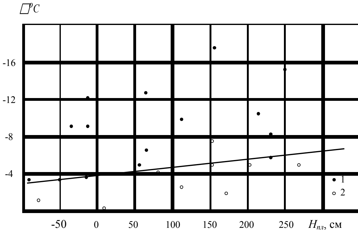
Рис.12.3 – Залежність t_{кр} = f(H_{л})
