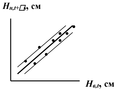
Рис.8.6 – Графік відповідних рівнів води при \Delta \neq \text{const}
