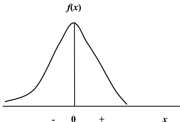
Рис.2.7 - Крива розподілу випадкової величини з від'ємною асиметрією (при C_S < 0 )
