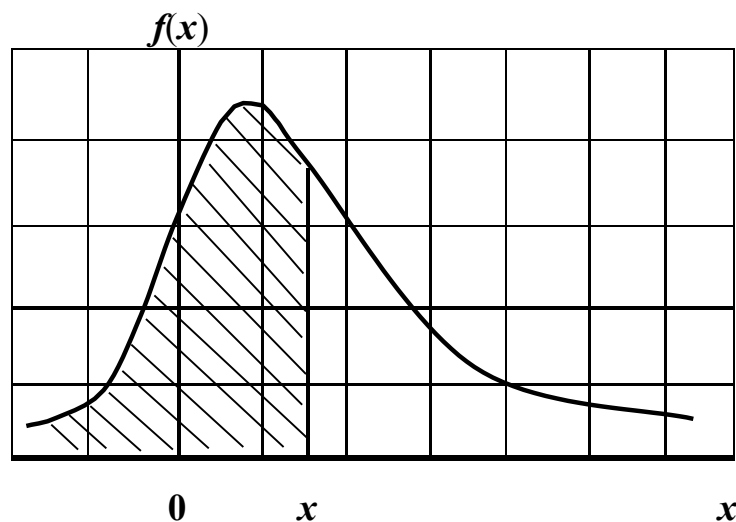
Рис. 2.4 - Крива розподілу випадкової величини x
