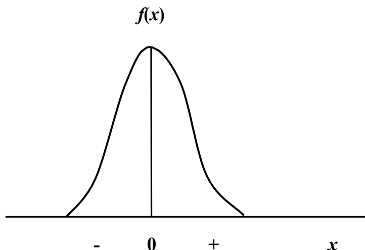
Рис.2.8 - Крива розподілу випадкової величини з симетричним розподілом (при C_S = 0 )
