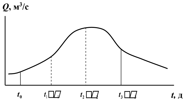
Рис. 8.3 – Гідрограф паводкової хвилі у нижньому створі припливної ділянки річки
