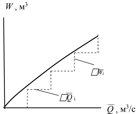
Рис. 9.7 – Визначення часу руслового добігання води на ділянці річки (при \square \neq const ) по кривій руслових запасів води
