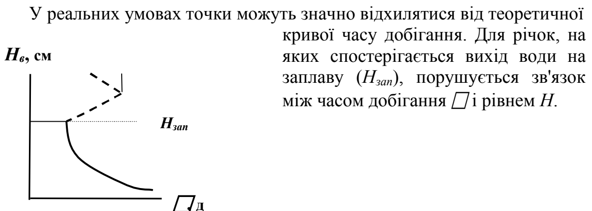
Рис.8.5- Графік часу добігання
