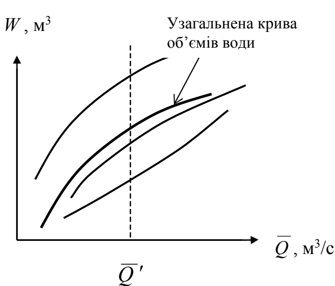
Рис. 9.4 – Побудова типової кривої руслових запасів води на ділянці річки
