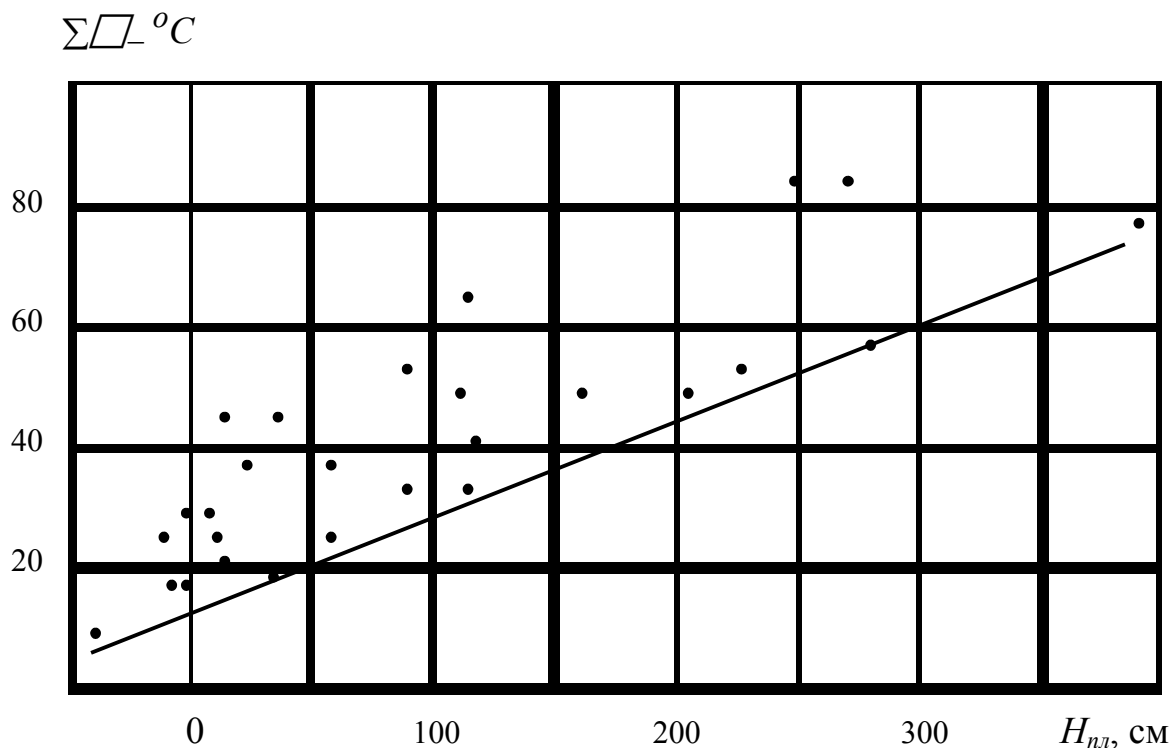
Рис.12.2 – Залежність \Sigma \square_{-min} = f(H_{нл}) .
