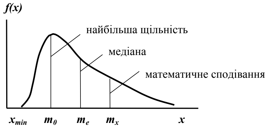
Рис. 2.5 - Крива розподілу з додатною асиметрією
