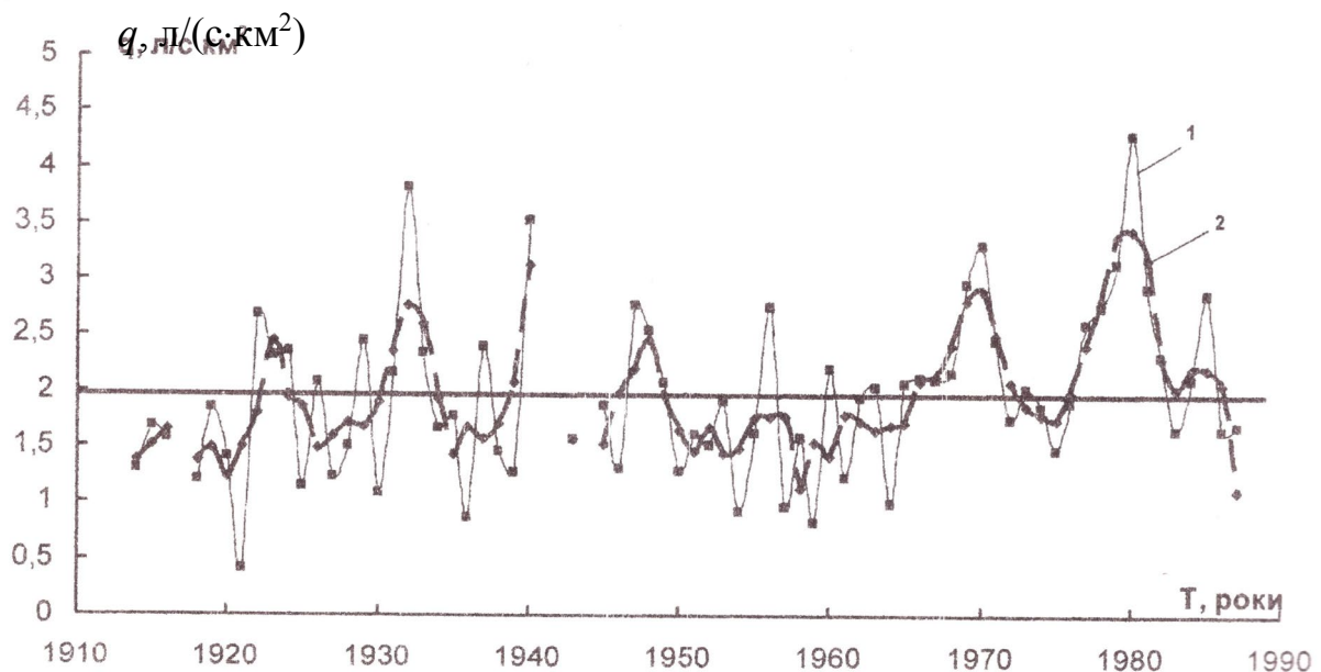
Рис.3.1 – Хронологічний графік коливань річного стоку (1) та графік згладжених середніх (2) р. Південний Буг – с. Олександрівка
