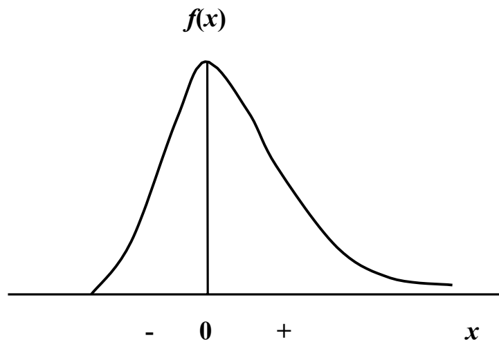
Рис. 2.6 - Крива розподілу випадкової величини з додатною асиметрією (при C_S > 0 )
