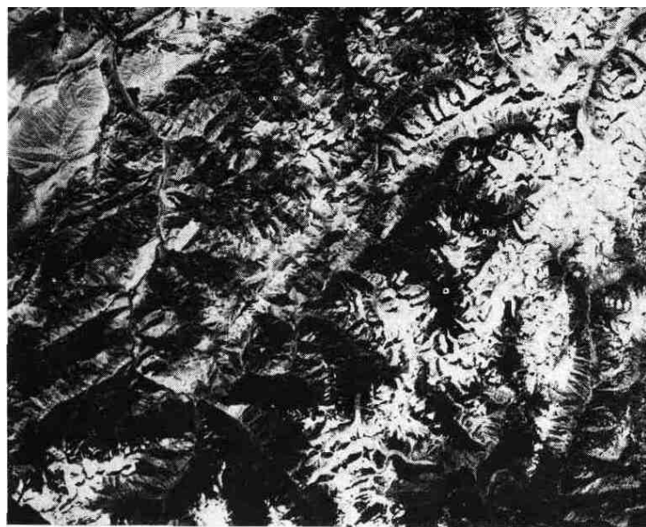
Рис. 1.4 – Дендритова текстура
