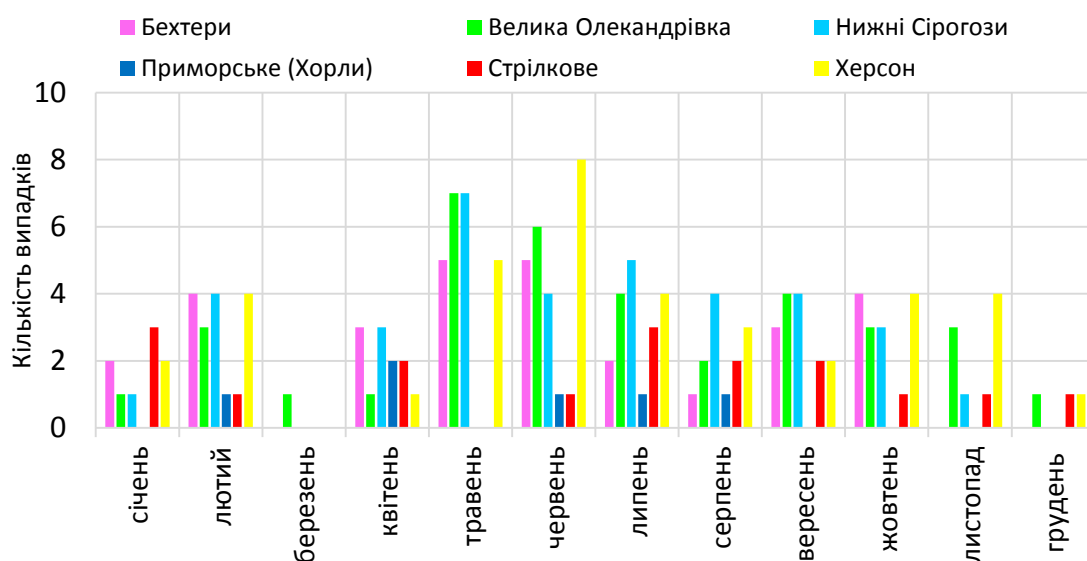
Рисунок 3 – Місячна повторюваність опадів на території Херсонській області за 2019-2020 рр.
