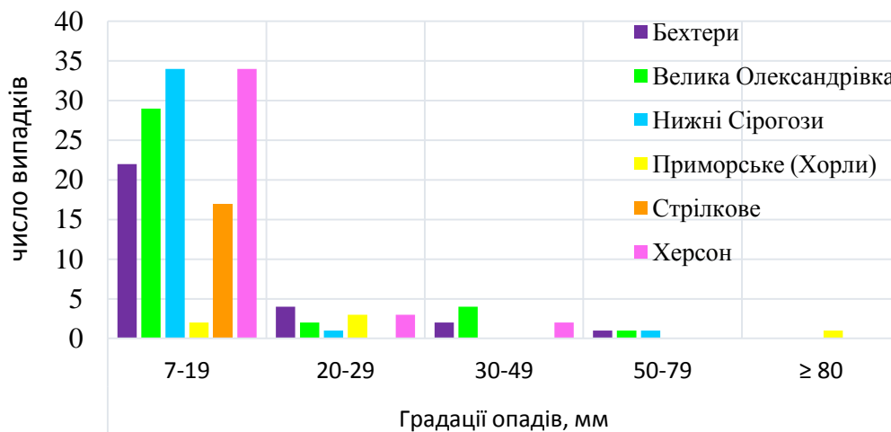
Рисунок 2 - Повторюваність опадів за градаціями на території Херсонській області за 2019-2020 рр.
