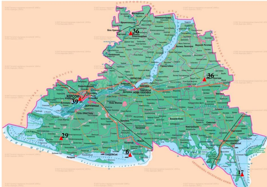
Рисунок 1 – Загальна повторюваність опадів \geq 7 мм по території Херсонської області, 2019-2020 рр.
