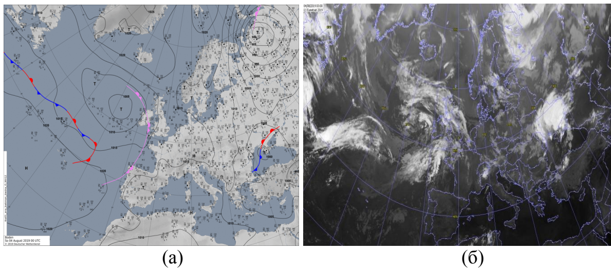
Рисунок 4 – Приземна карта погоди 04.08.2019 р., 00 UTC – (а); супутниковий знімок хмарності, 03:00 UTC – (б)
