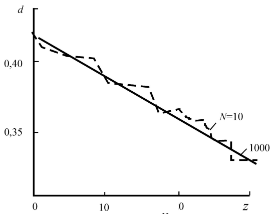
Рис. 5.2. Залежність ймовірності d простоювання складального цеху від розміру страхового запасу Z_c^H при різних значеннях числа дублювань спроб N
