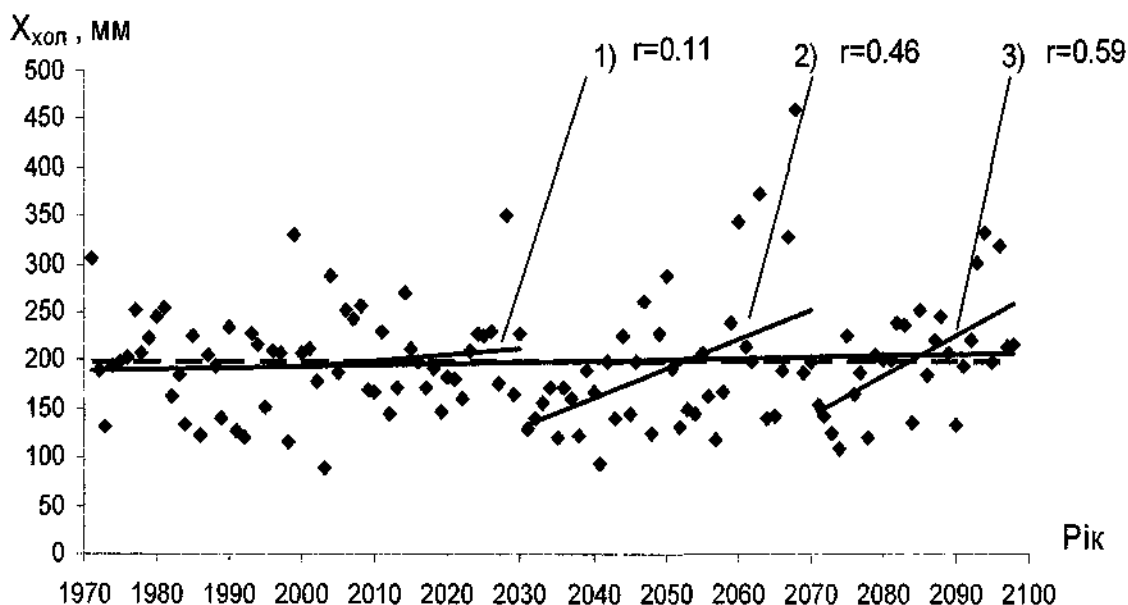
Рис. 6. Хронологічний хід сум опадів холодного (XI-III міс.) періоду, точка №4, 1971-2098 рр. (---- середнє багаторічне значення, ——— лінія тренду, 1 – 2001-2030 рр., 2 – 2031-2070 рр., 2071-2098 рр.)
