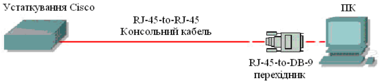
Рисунок В.3 – Схема підключення до консольного інтерфейсу
