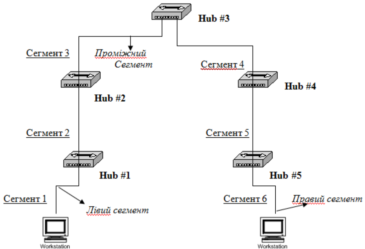
Рис.4.12 – Конфігурація мережі Ethernet
