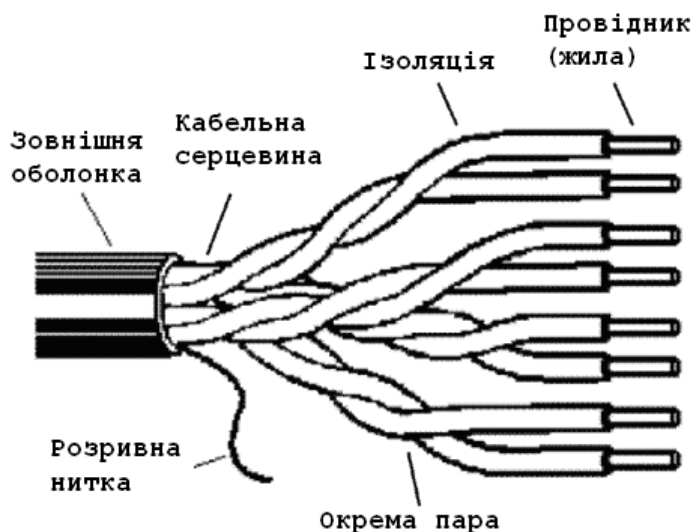
Рис. 4.10 - Кабель «кручена пара»
