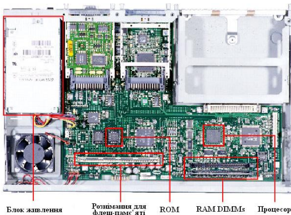
Рисунок В.1 – Внутрішні компоненти Cisco Router 2600
