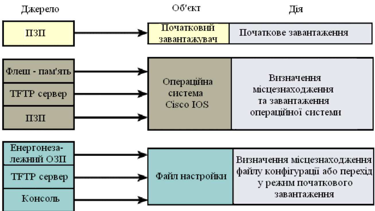
Рисунок Г.1 – Послідовність завантаження Cisco IOS
