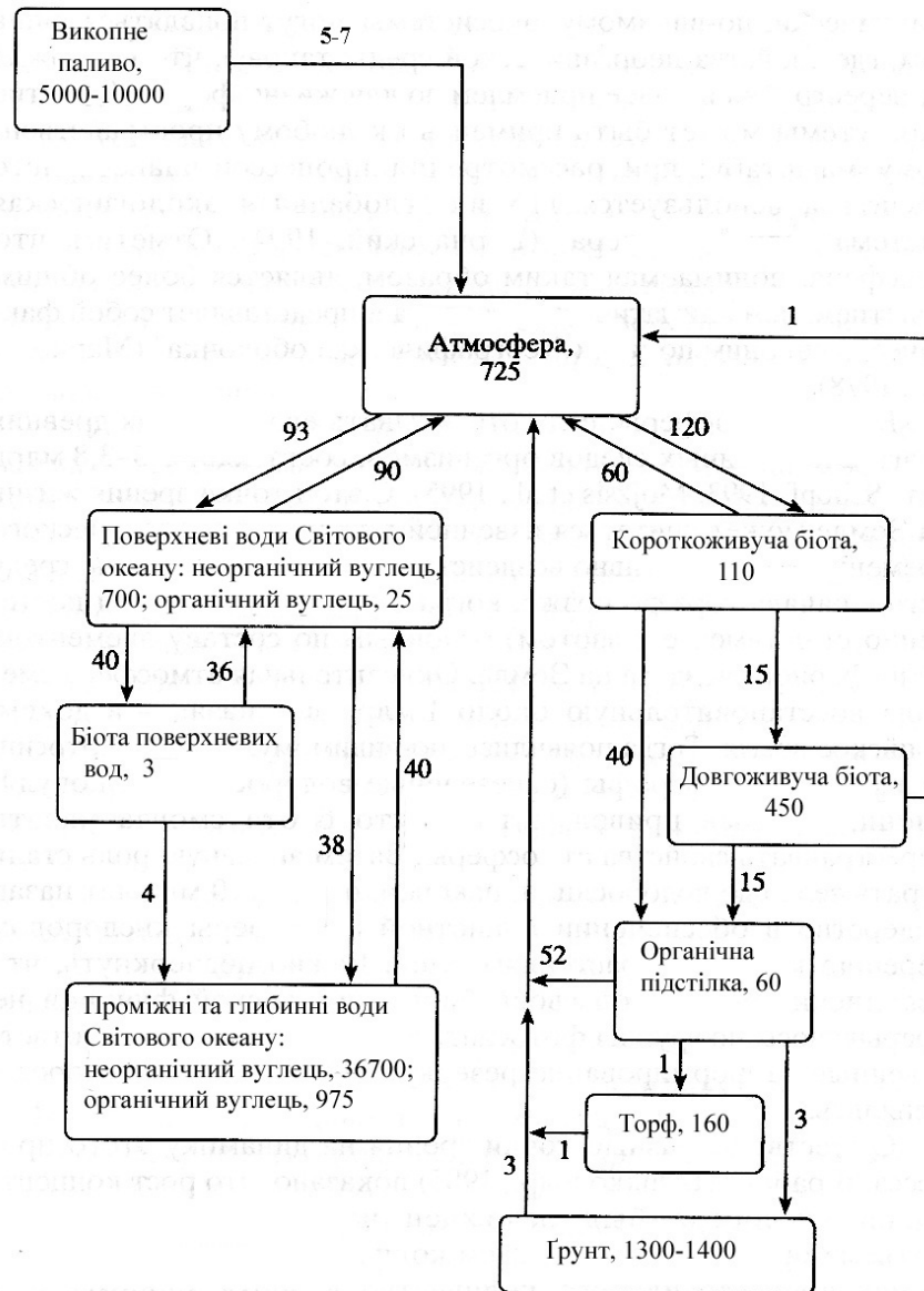
Рисунок 10.30 – Блок-схема глобального циклу вуглецю (Кислов, 2001). Вміст вуглецю наведений у 10^{12} кг, потоки між резервуарами – в 10^{12} кг/рік.
