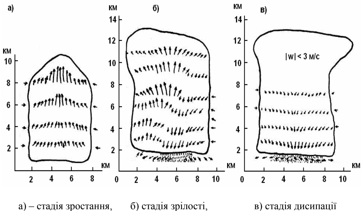
Рисунок 8.1 – Еволюція Св (за Байерсом та Брейамом)
