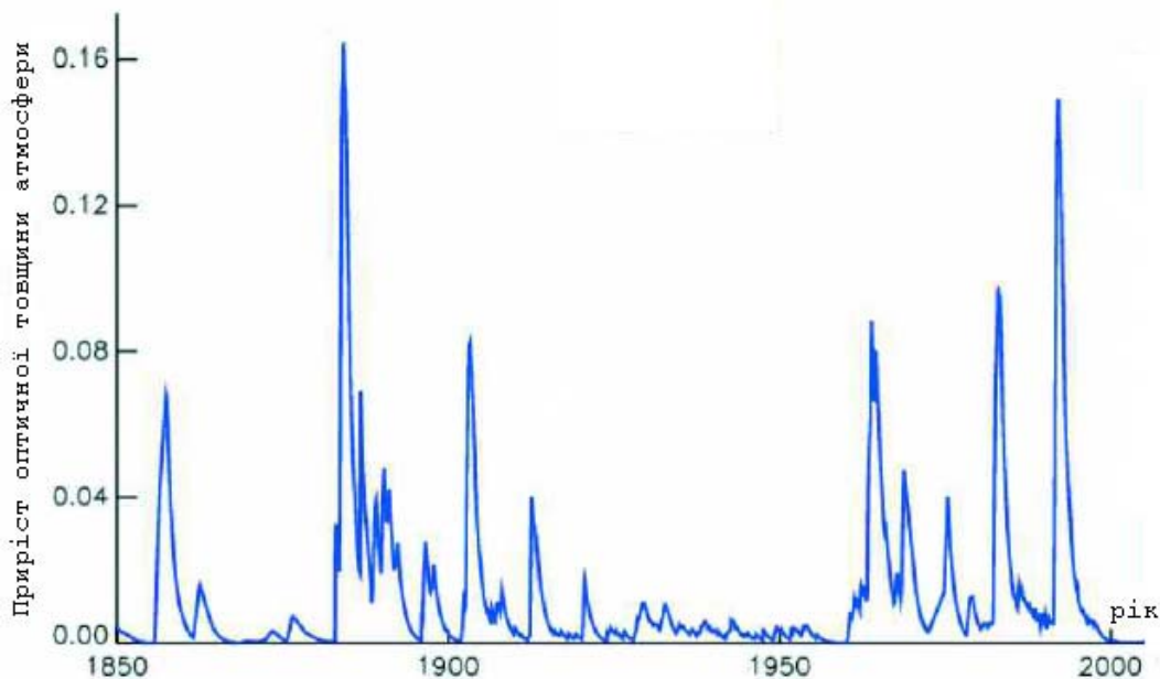
Рисунок 10.28 – Зміни оптичної товщини атмосфери (на хвилі 5 мкм), обумовлені викидами аерозолів у стратосферу за рахунок вулканічної діяльності (Climate Change 2007)
