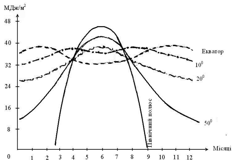
Рисунок 10.5 – Річний хід добової інсоляції на верхній межі атмосфери для Північної півкулі
