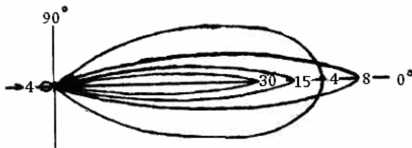
Рисунок 5.12 – Індикатриса розсіювання радіації краплями води (цифри на кривих характеризують значення параметра \mu = 2\pi x/\lambda )
