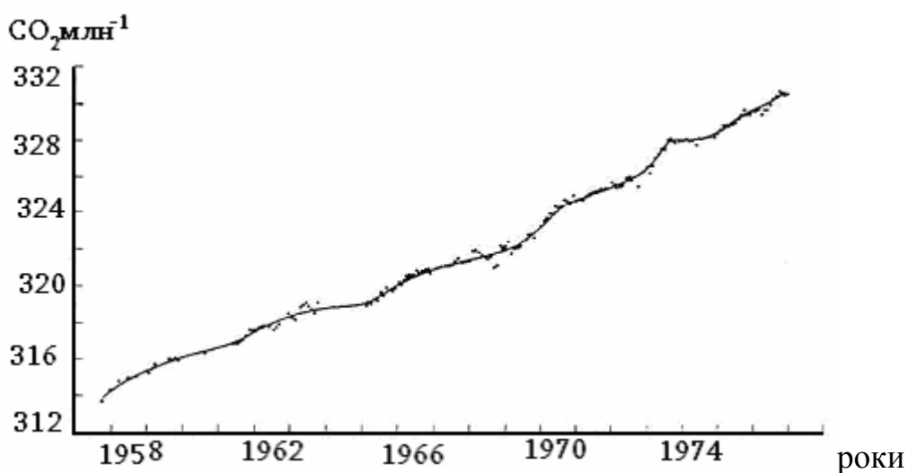
Рисунок 1.4 – Осереднена по сезонах концентрація \text{CO}_2 на Південному полюсі
