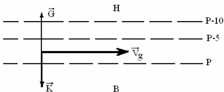
Рисунок 7.1 – Взаємне розташування векторів геострофічної швидкості \vec{V}_g , сил горизонтального баричного градієнта \vec{G} і Кориоліса \vec{K} у випадку геострофічного руху
