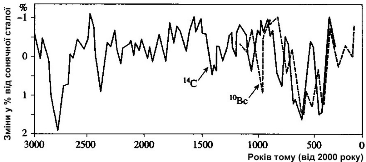
Рисунок 10.22 – Реконструйовані часові варіації сонячної сталі за останні 3 тис. років (Кислов, 2001)
