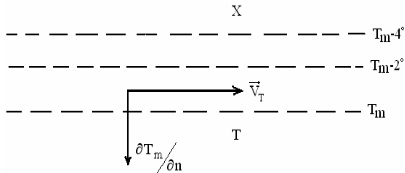
Рисунок 7.2 – Взаємне розташування векторів швидкості термічного вітру \vec{V}_T і градієнта середньої температури шару \frac{\partial \bar{T}_m}{\partial n}
