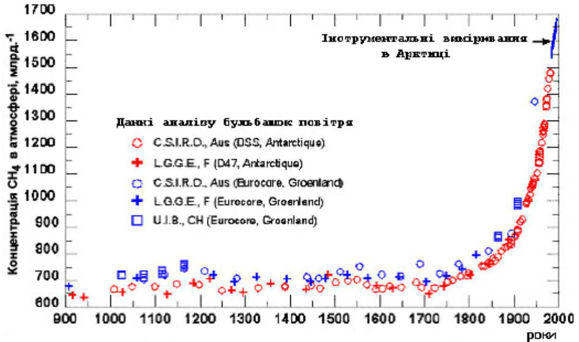
Рисунок 10.33 – Зміни концентрації метану в атмосфері з 900 по 2000 рік нашої ери за даними аналізу бульбашок повітря, які залишилися у льоду Антарктиди та Гренландії, а також інструментальних вимірювань на арктичних полярних станціях (Рис. з сайту www-lgge.ujf-grenoble.fr )
