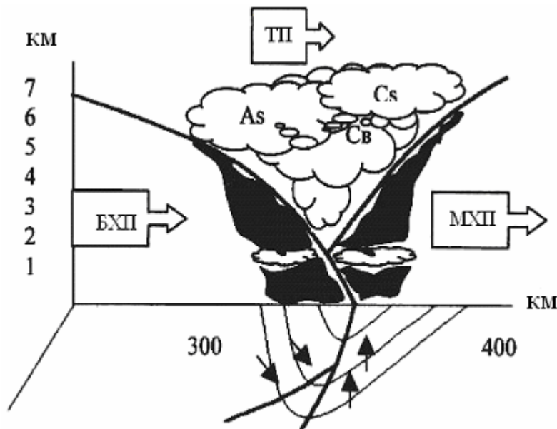
Рисунок 9.2 – Схема фронту оклюзії
