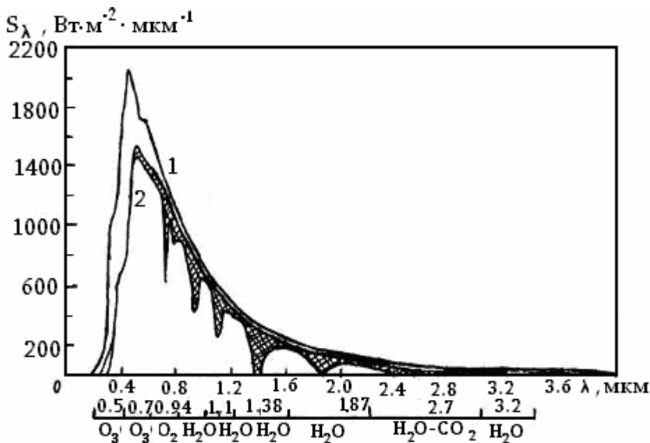
Рисунок 5.7 – Розподіл спектральної щільності потоку сонячної радіації
