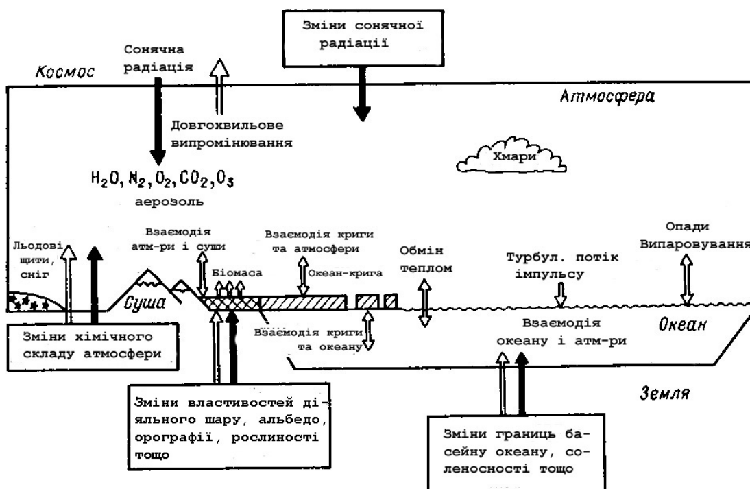
Рисунок 10.3 – Спрощена схема взаємодії компонентів глобальної кліматичної системи (Глобальный климат, 1987)
