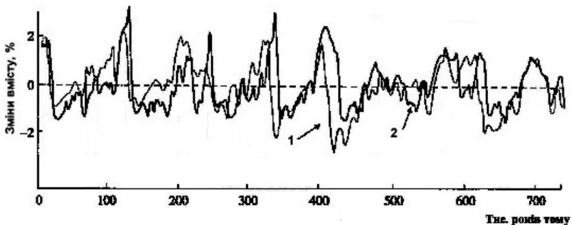
Рисунок 10.37 – Відносні зміни вмісту важкого ізотопу кисню \delta^{18}\text{O} (1 - станція „GeoB1413”) та дейтерію \delta\text{D} (2 - станція „Купол С”) за останні 750 тис. років (Вакуленко, 2007).
