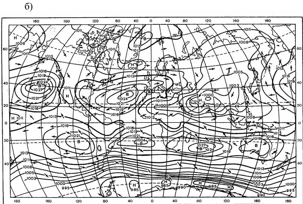
Рисунок 10.11 – а) Повторюваність (%) рухомих циклонів. Липень; б) Середнє поле атмосферного тиску (гПа) та течії повітря на рівні моря. Липень. (Клімат України, 2003)
