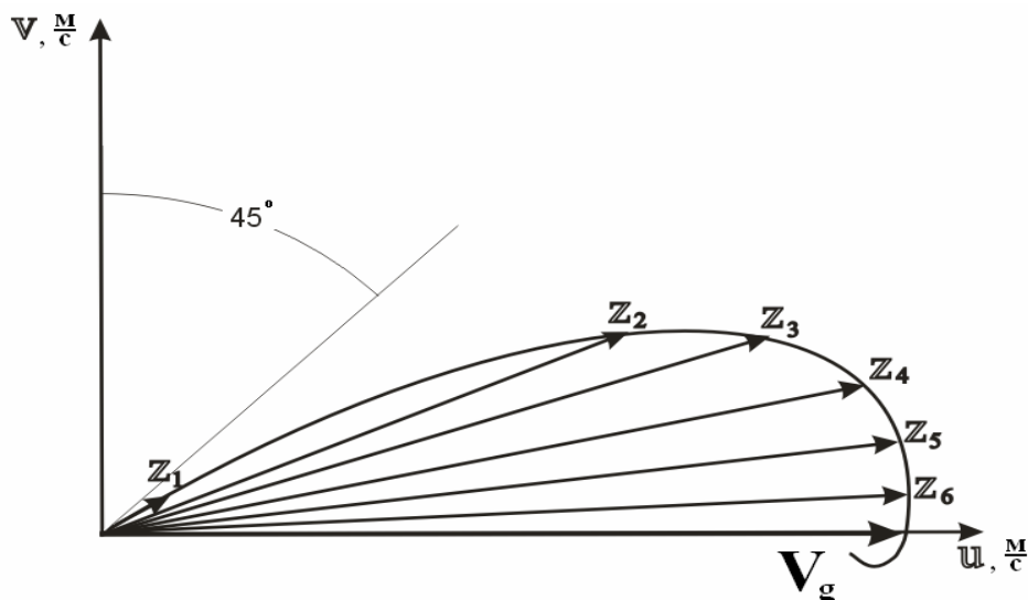
Рисунок 7.8 – Годограф швидкості вітру у граничному шарі
