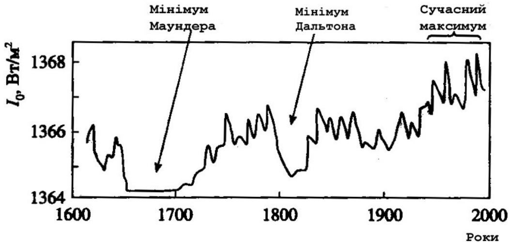
Рис. 10.23 – Реконструйовані часові варіації сонячної сталої за останні 400 років (Кислов, 2001)
