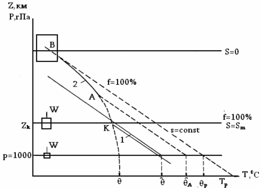
1 – суха адіабата, 2 – волога адіабата, z_k – рівень конденсації, ОКAB – крива стану частинки повітря
