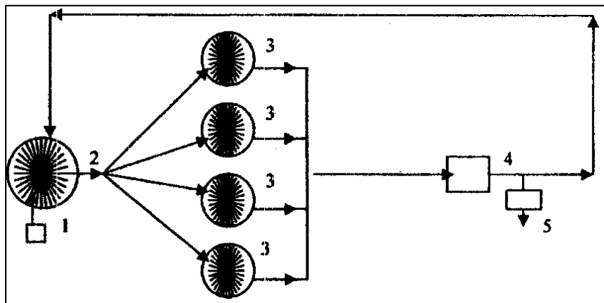
Рис. 1 – Схема лабораторной установки для исследования биохимических процессов очистки воды иммобилизованными анаэробными микроорганизмами
