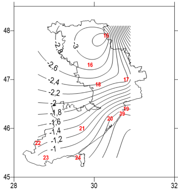
Рисунок 2.9 – Поле середніх значень температури повітря в січні на станціях Одеської області
