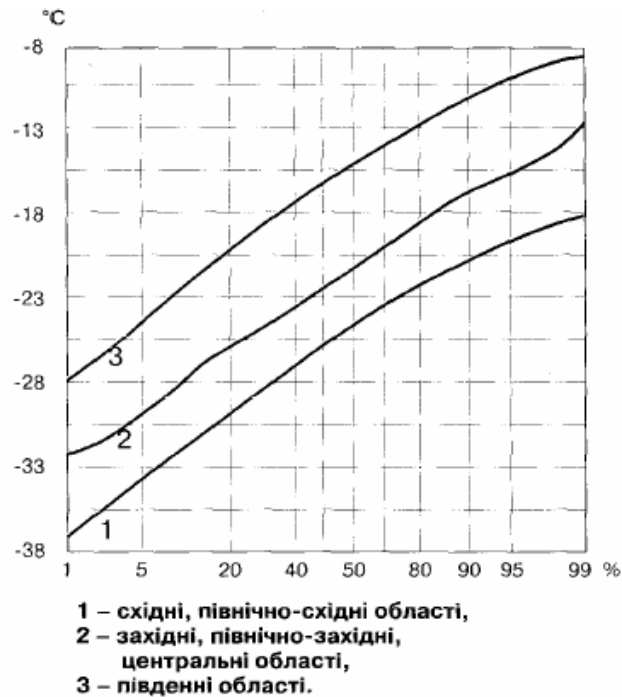
Рисунок 1.17 - Абсолютний мінімум температури повітря °С різної ймовірності (%) рівний та вищий вказаних значень в окремих районах [1]
