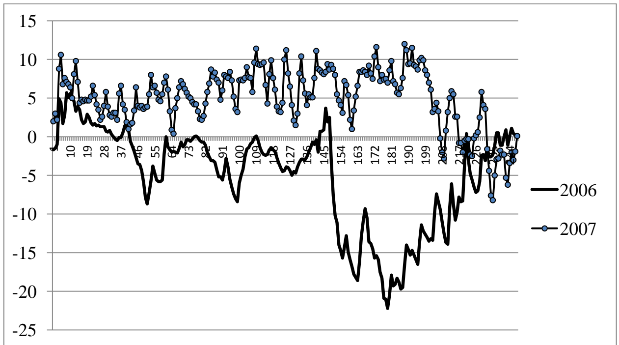
Рис. 2.7 – Часові ряди температури повітря строкових спостережень в січні на станції Одеса (2006 та 2007 роках)
