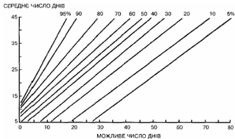
Рисунок 1.14 - Номограма для розрахунку числа днів з температурою повітря -10\text{ }^{\circ}\text{C} нижче різної ймовірності (%) рівне та вище вказаних значень. Рік [1]
