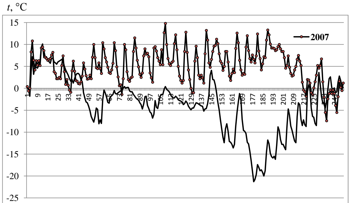
Рис. 2.5 – Часові ряди температури повітря строкових спостережень в січні на станції Вілково (2006 та 2007 роках)
