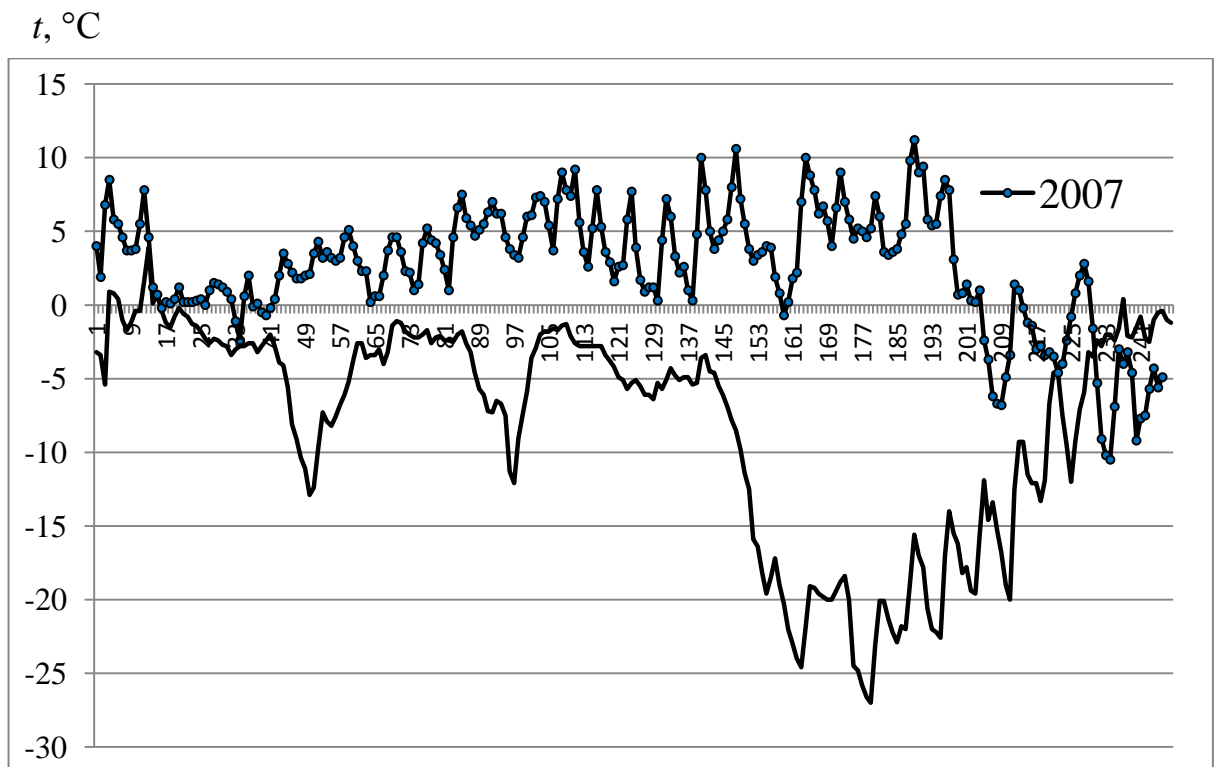
Рис. 2.6 – Часові ряди температури повітря строкових спостережень в січні на станції Любашівка (2006 та 2007 роках)
