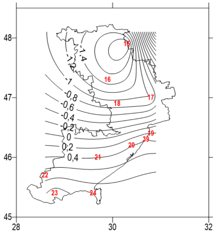
Рисунок 2.9 – Поле середніх значень температури повітря в січні на станціях Одеської області
