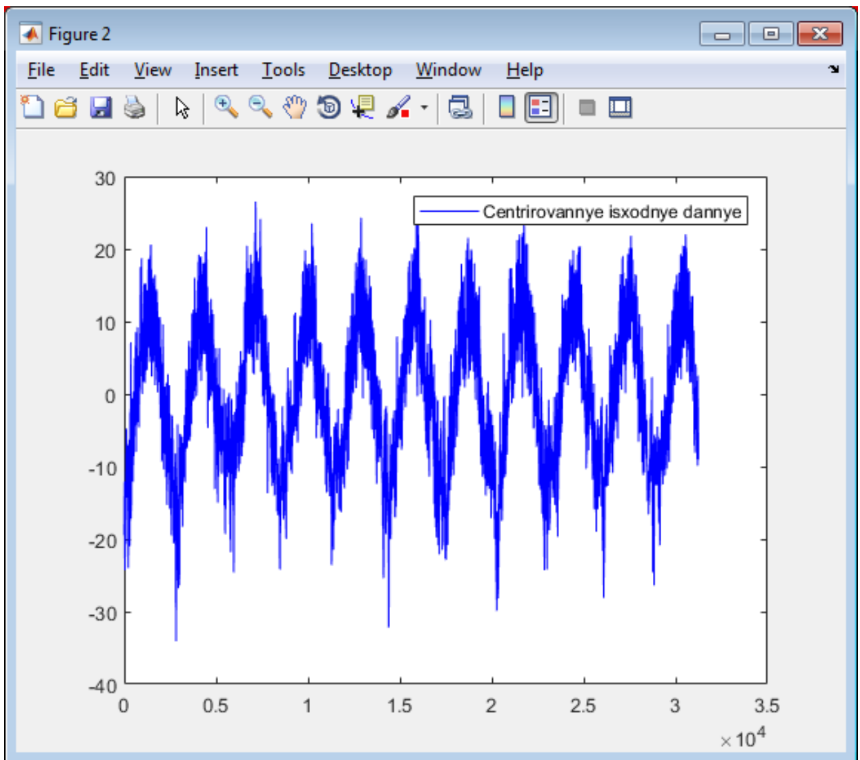
Рисунок 4.6 – Графік центрованих вхідних даних
