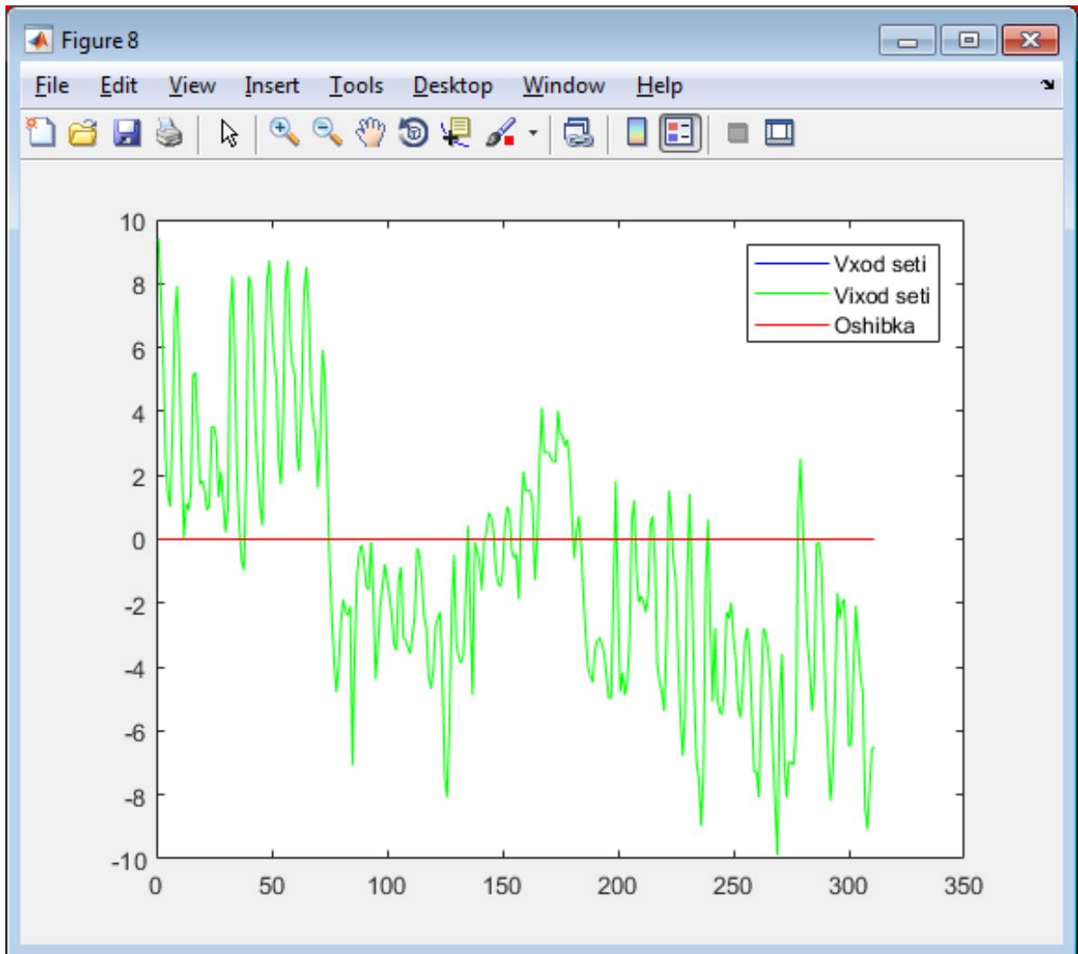
Рисунок 4.9 – Графік входу, виходу та похибки на центрованому ряді температур
