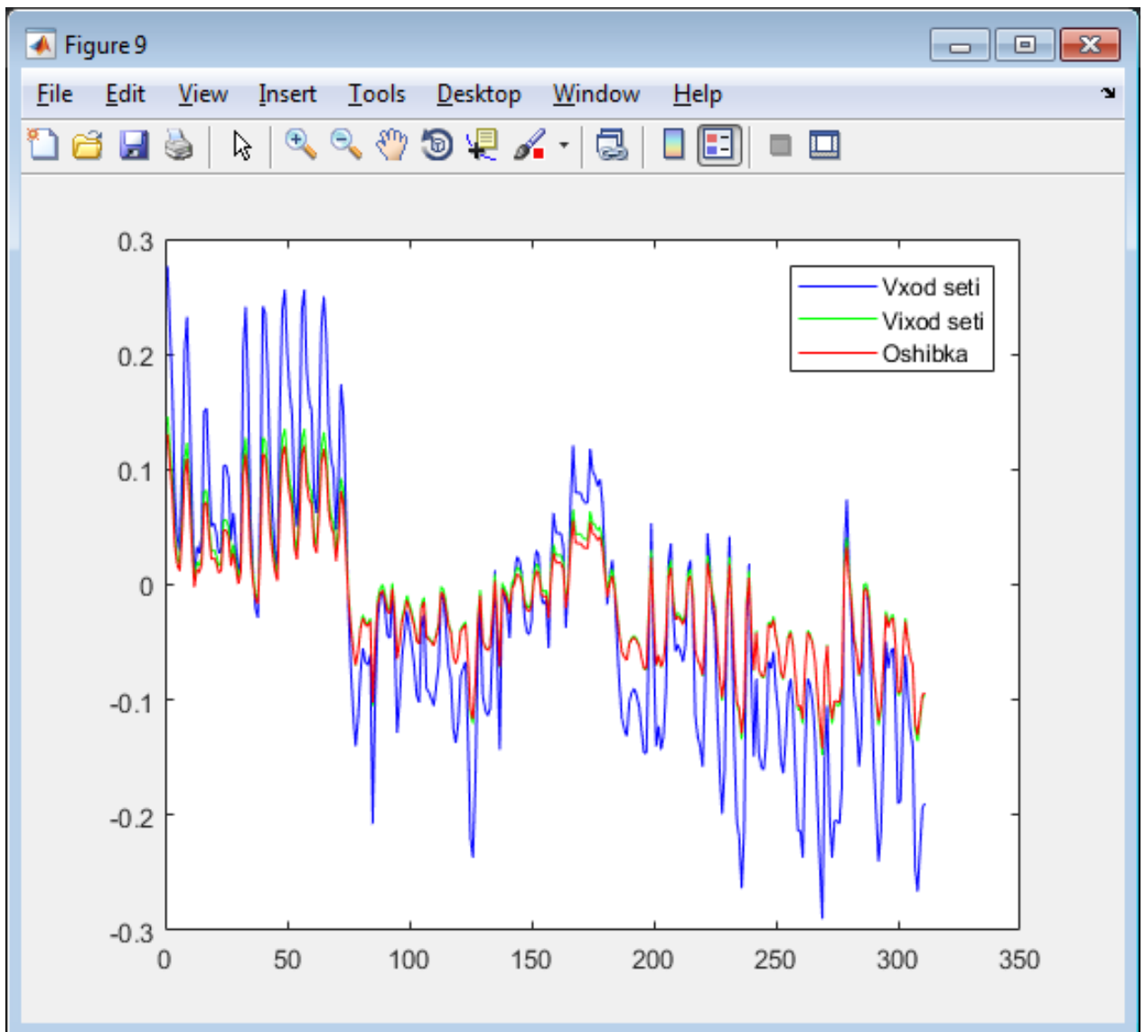
Рисунок 4.13 – Графік входу, виходу та похибки на центровано-нормованому ряді температур
