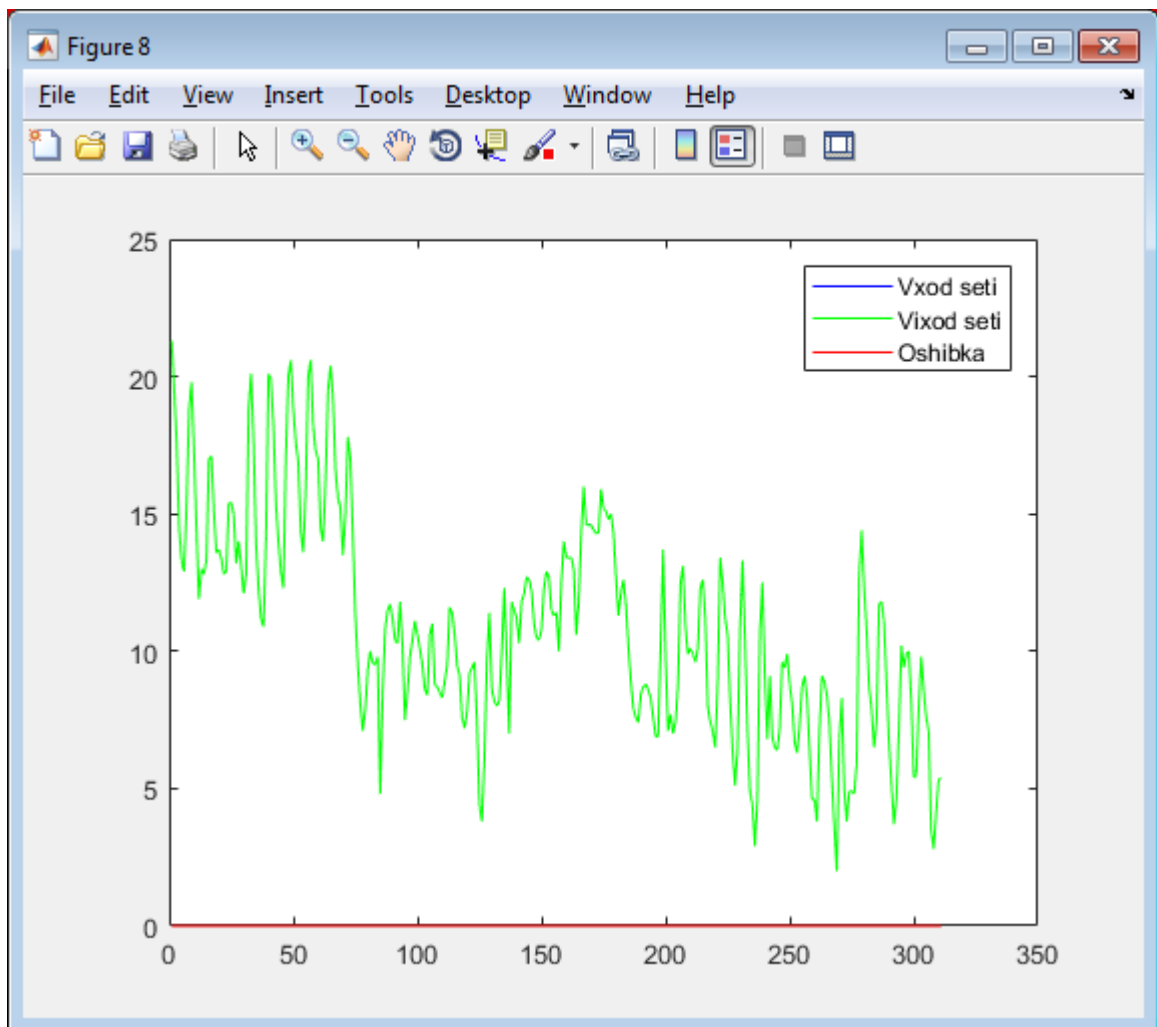
Рисунок 4.4 – Графік залежності входу мережі, виходу та похибки
