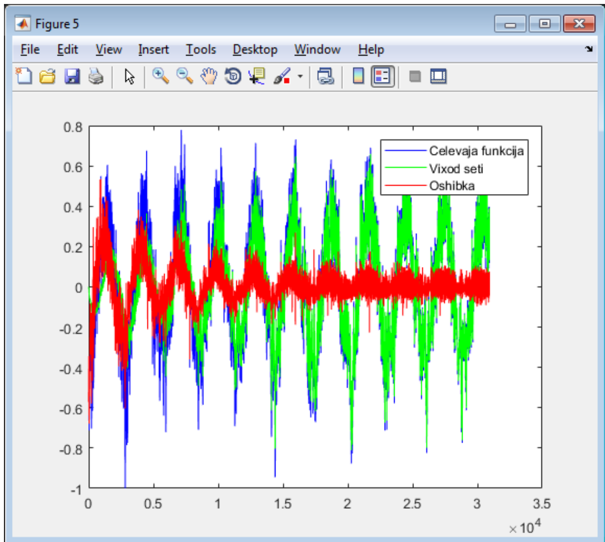
Рисунок 4.12 – Графік залежності похибки та виходу мережі з цільовою функцією
