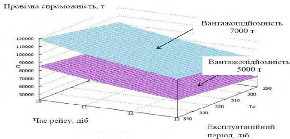
Рисунок 2 – Зміна провізної спроможності для суден-мінібалкерів з чистою вантажопідйомністю 5000 т і 7000 т при зміні експлуатаційного періоду та часу рейсу судна
