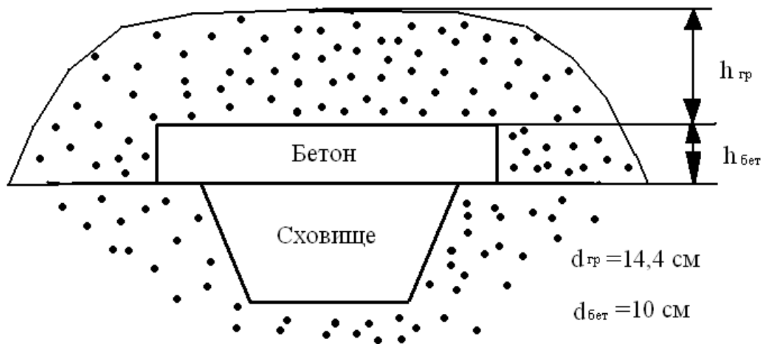
Рис. 1.2 – Схема визначення параметрів, по яким розраховуються коефіцієнтів ослаблення для сховища.
