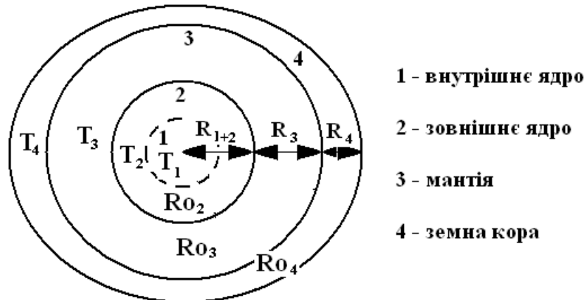
Рис. 1.1 – Внутрішня структура земної кулі. R ( R_{1+2}=3400 км, R_3=2950 км, R_4=5-70 км) – радіуси зон; T ( T_1=5000 °C, T_2=4000 °C, T_3=1000-3500 °C) – температура в зонах; R_0 ( R_{01}=14 г/см 3 , R_{02}=10 г/см 3 , R_{03}=(3 \dots 10) г/см 3 , R_{04}=2,9 \dots 2,6 г/см 3 ) – густина в зоні.
